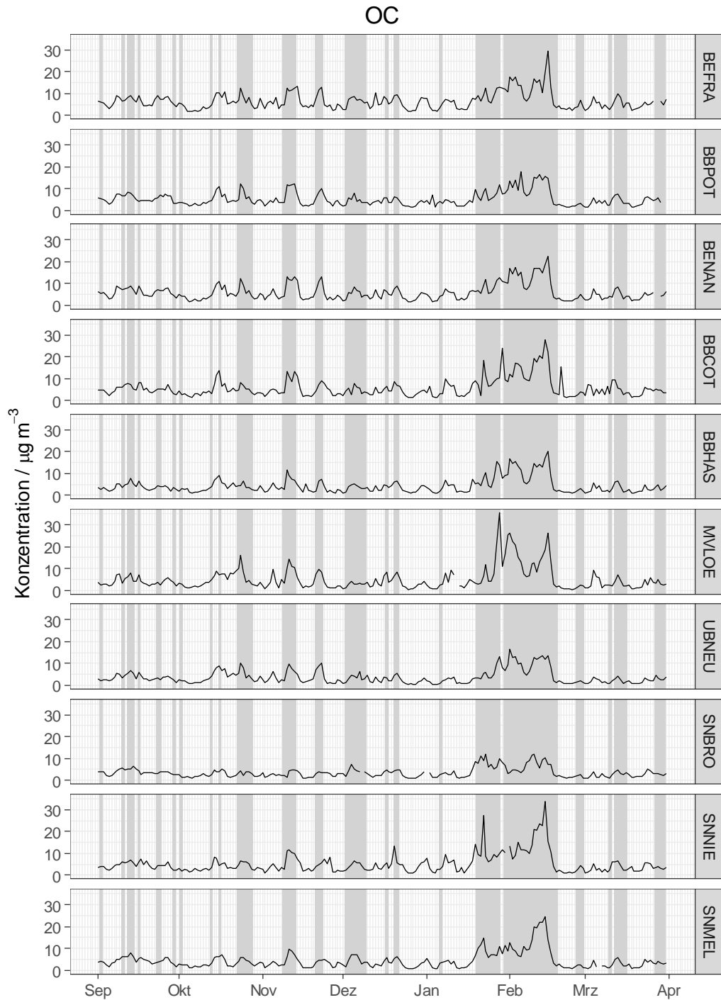
Abbildung 16: Tägliche Konzentration von OC im PM10 für die einzelnen Messstationen im Untersuchungszeitraum; SMT grau hinterlegt.
