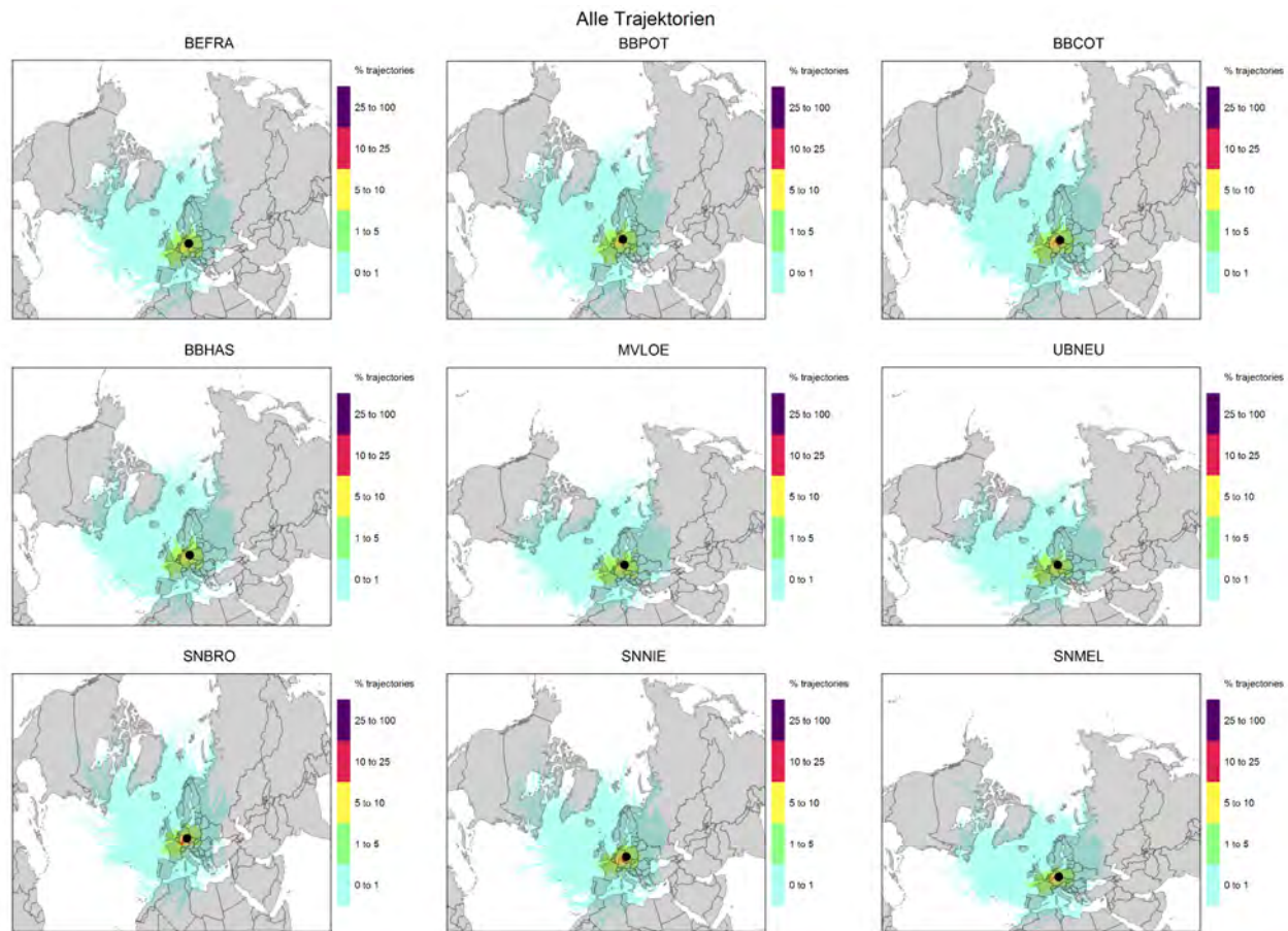
Abbildung 2: Geographische Häufigkeitsverteilung für alle 96h- Rückwärtstrajektorien im Untersuchungszeitraum. Auf die Darstellung der Messstation BENAN wurde aufgrund der lokalen Nähe zur Messstation BEFRA verzichtet.
