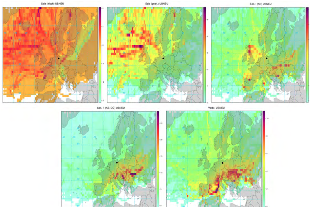
Abbildung 63: CWT Plots für Quellbeiträge PMF für die Station UBNEU. Von links oben nach rechts unten sind gezeigt: Salz (frisch), Salz (gealtert), sekundäres Ammoniumnitrat, sekundäres Ammoniumsulfat und OC, Aerosol aus Verbrennung. Die negativen Zahlen an der Ordinate für Salz (frisch) oben links entstehen dadurch, dass die PMF dem Sulfat negative Konzentrationen zuordnet.
