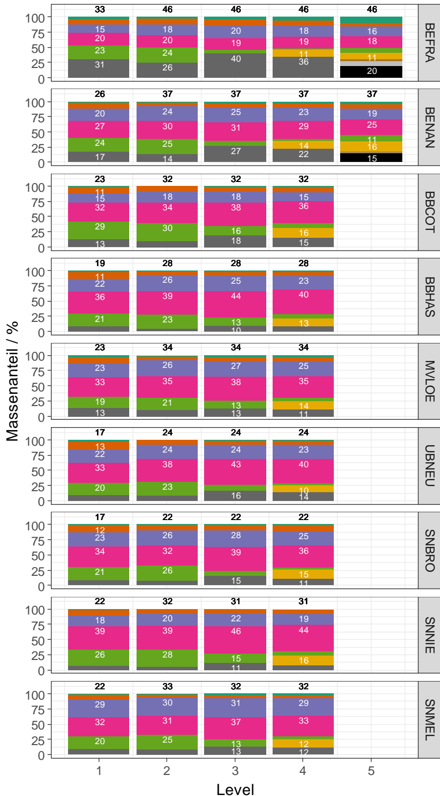
Abbildung 62: Übersicht über die relativen Beiträge verschiedener Quellkategorien zur PM 10 -Gesamtkonzentration für die PMF Level 1 – 5 und für die verschiedenen Messstationen.
