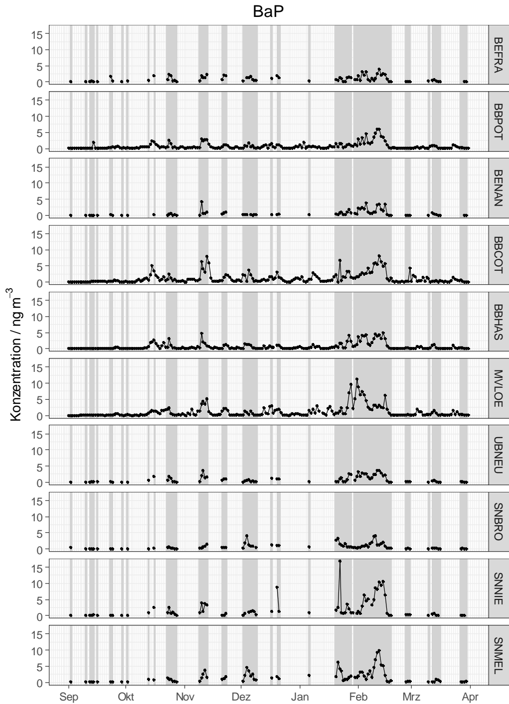
Abbildung 23: Tägliche Konzentration von Benzo(a)pyren im PM10 für die einzelnen Messstationen im Untersuchungszeitraum; SMT grau hinterlegt.
