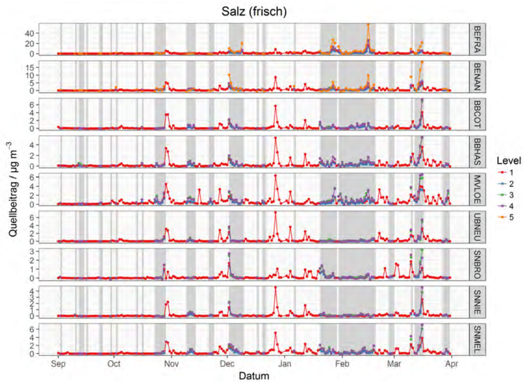
Abbildung 51: Zeitreihen der PMF-modellierten Quellbeiträge für den Faktor frisches Salz im direkten Vergleich der 5 PMF Levels.
