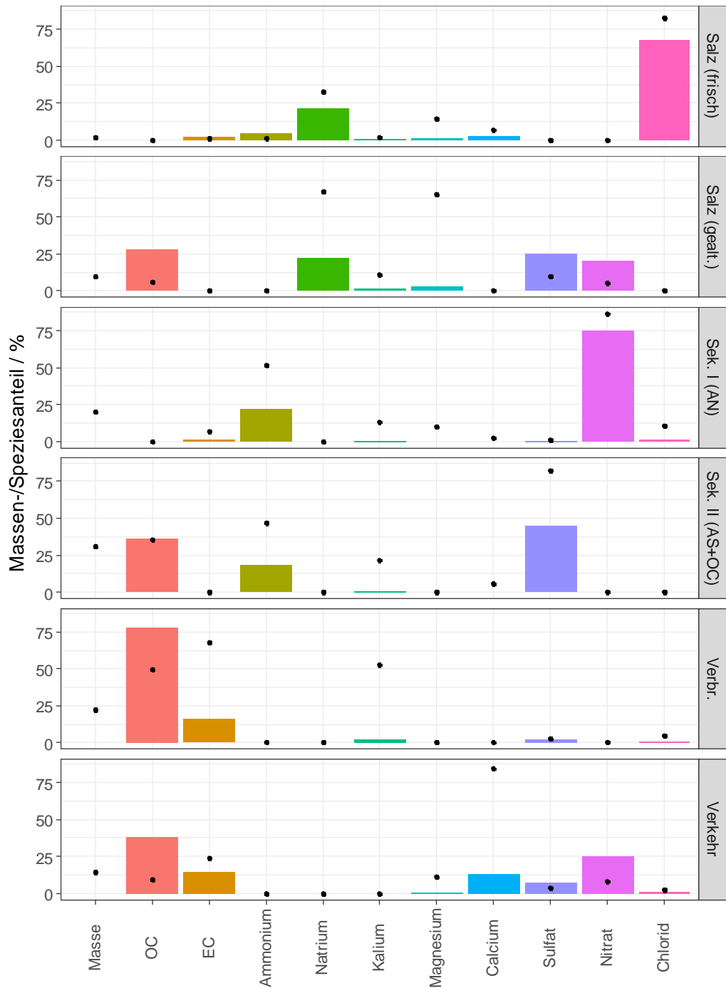
Abbildung 45: Quellprofile der 6 Faktoren des Level 1 PMF Laufes. Balken geben den Massenanteil in % der Faktormasse an (Summe aller Verbindungen im Faktor = 100%), Punkte den Speziesanteil in % der Gesamt-Spezieskonzentration (Summe der Spezies über alle Faktoren = 100%).
