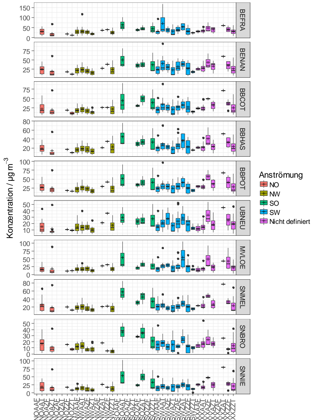
Abbildung 33: PM10- Massekonzentration in Abhängigkeit von den Wetterlagenklassen nach OWTC und Eingruppierung nach dem Windindex für 700 hPa für alle 10 Messstationen.
