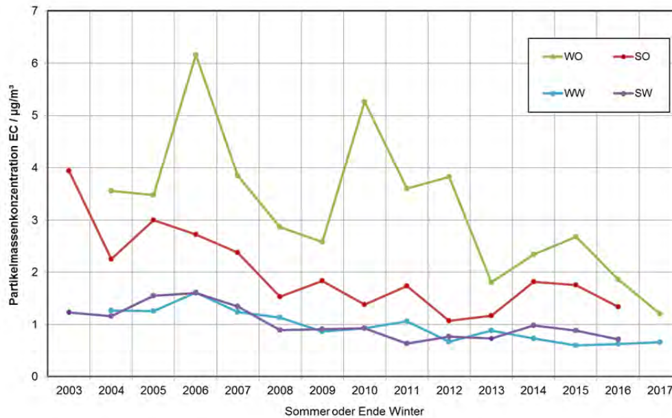
Abbildung 18: Jahreszeitenmittel für EC (Sommer und Winter), Einordnung nach Anströmung (Ost/West) und Jahreszeit (Sommer/Winter) AIWE, vergleiche Kapitel 2.4.1. Für 2015, 16 und 17 wurden die EC- Konzentrationen für das thermographische Verfahren nach VDI ausgehend vom thermooptischen Verfahren (Temperaturprotokoll EUSAAR2 und Transmission) abgeschätzt. Für den Winter 2016/17 im Projektzeitraum wurden nur 5 Monate (NDJFM) gemittelt.
