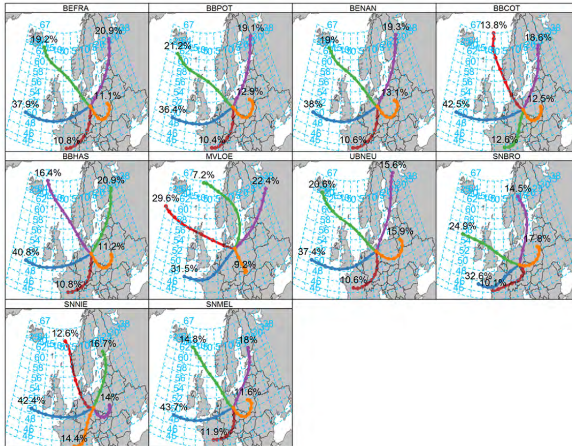
Abbildung 42: Überblick über das Ergebnis der separaten Clusteranalyse für jede der 10 Stationen im Untersuchungsgebiet mit jeweils 5 Clustern. Die Farben der Trajektoriencluster weichen hier teilweise im Vergleich zu Abbildung 40 ab.
