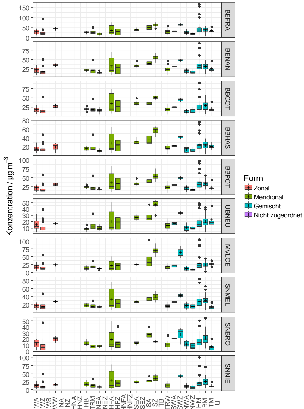
Abbildung 34: PM10- Massekonzentration in Abhängigkeit von den Wetterlagenklassen nach SHBC und Eingruppierung nach Zirkulationsform für alle 10 Messstationen.
