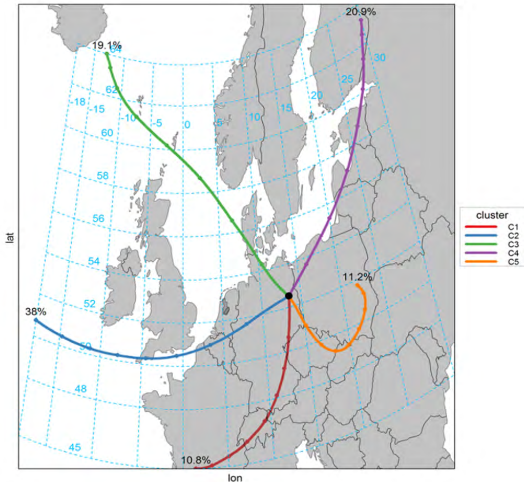
Abbildung 40: Clusteranalyse für die Station BEFRA im Untersuchungszeitraum mit den Clustern:
