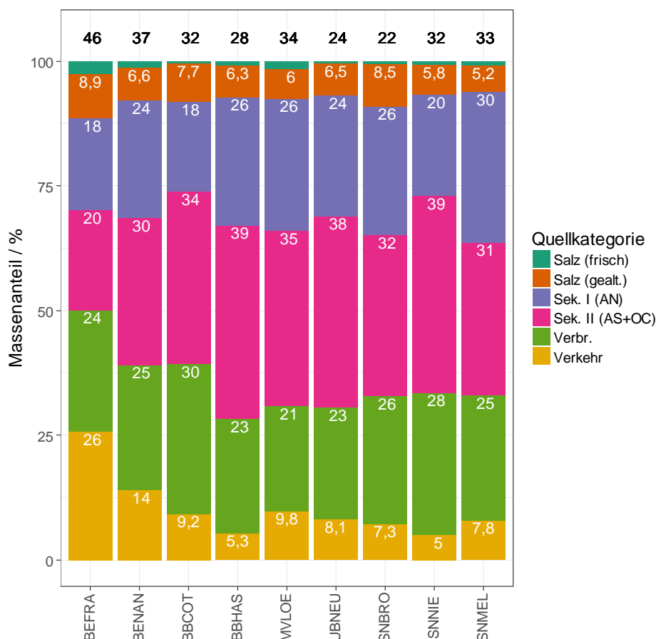
Abbildung 59: Anteile der auf PMF Level 2 identifizierten Quellkategorien an der mittleren PM10- Massekonzentration (schwarze Zahlen über Balken) der Stationen.
