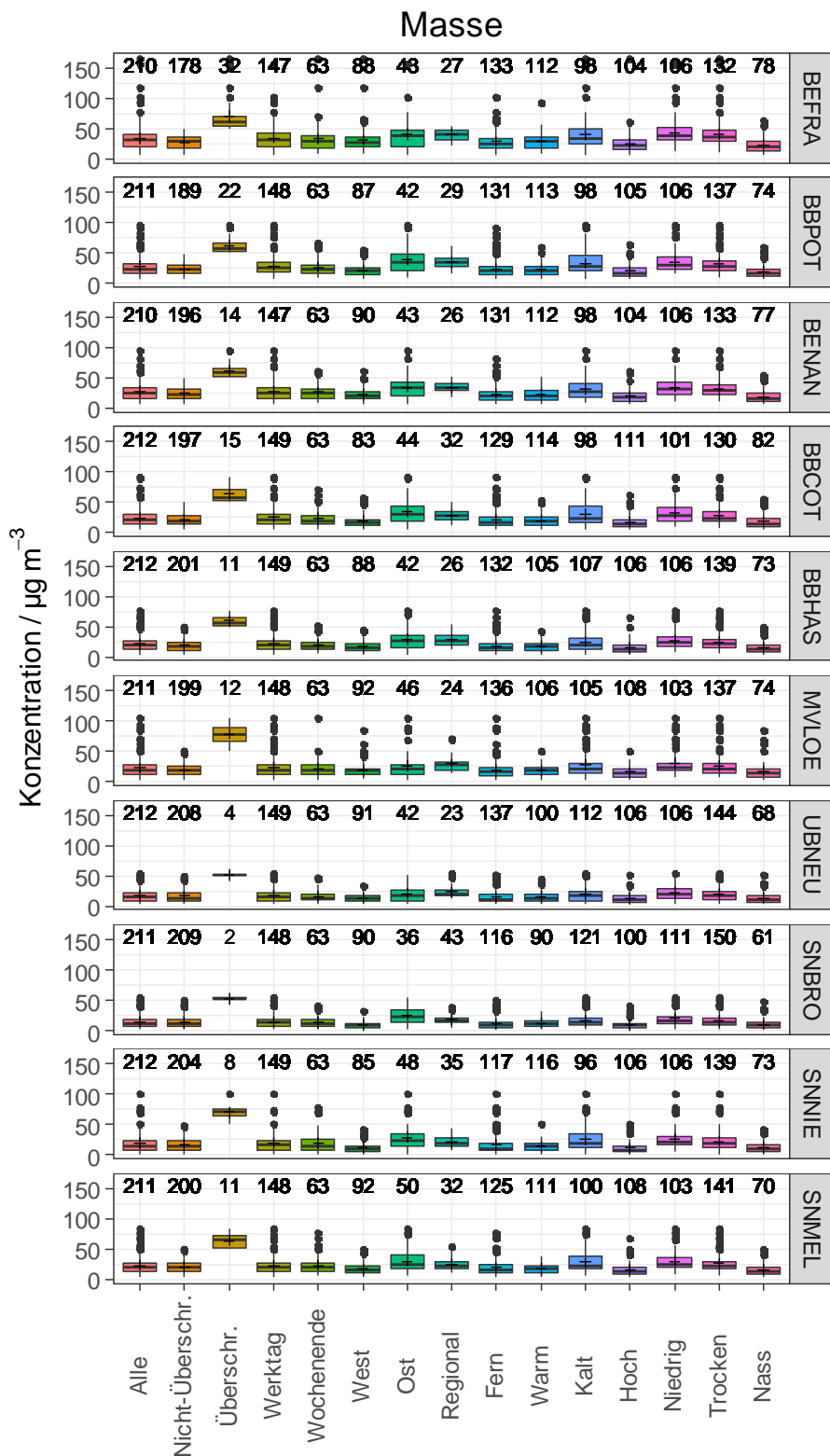
Abbildung 24: PM10- Massekonzentration für alle Messtage und in Abhängigkeit von der Tagescharakteristik und den Belastungskategorien für alle 10 Messstationen. Die Zahlen über den Boxen kennzeichnen die Anzahl der verfügbaren Messwerte.
