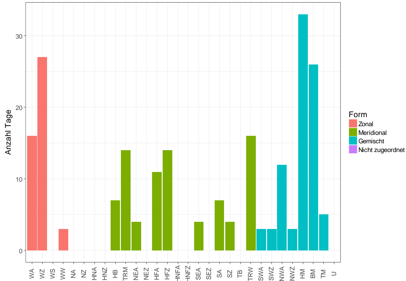
Abbildung 12: Anzahl der Messtage in den Wetterlagenklassen nach SHBC und Eingruppierung nach Zirkulationsform.
