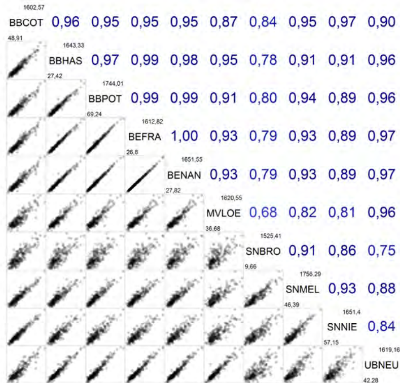
Abbildung 9: Korrelationsmatrix für die Mischungsschichthöhe aus dem COSMO-CLM Modell zwischen den Stationen.
