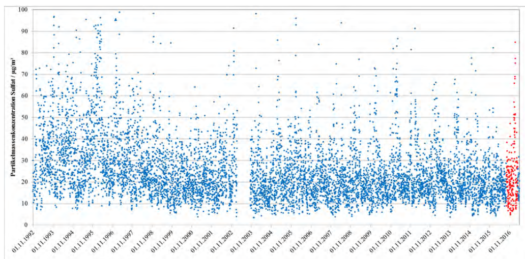
Abbildung 14: Verlauf der täglichen PM10- Massekonzentration an der Station SNMEL seit 1992. Die Ergebnisse der 212 Tage des PM-OST Projektes sind in rot gezeigt.
