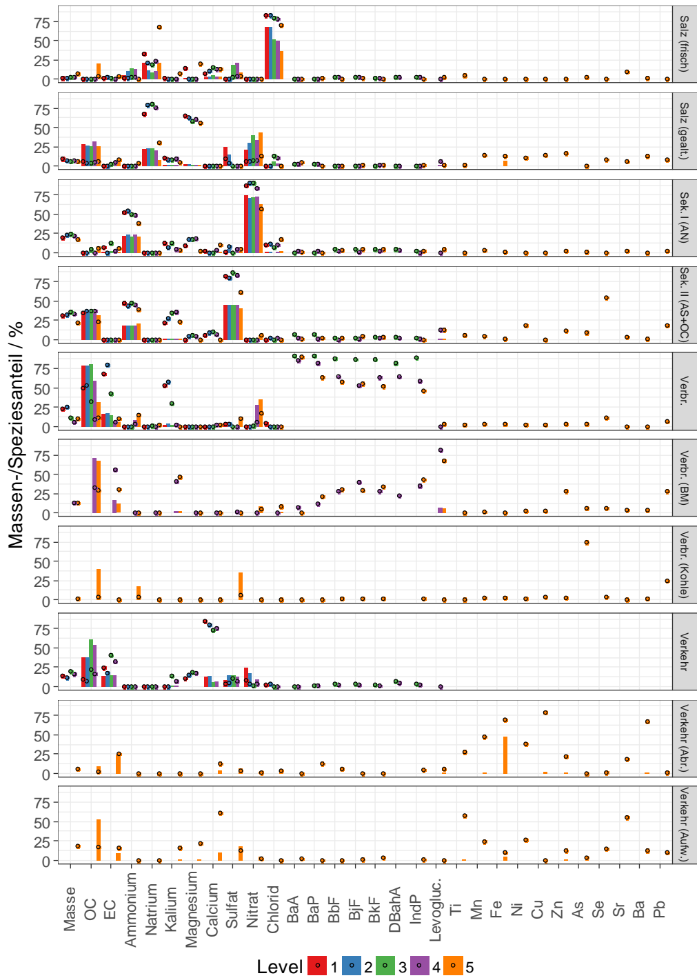
Abbildung 50: Quellprofile aller PMF-Faktoren in den Levels 1 – 5 im Vergleich.
