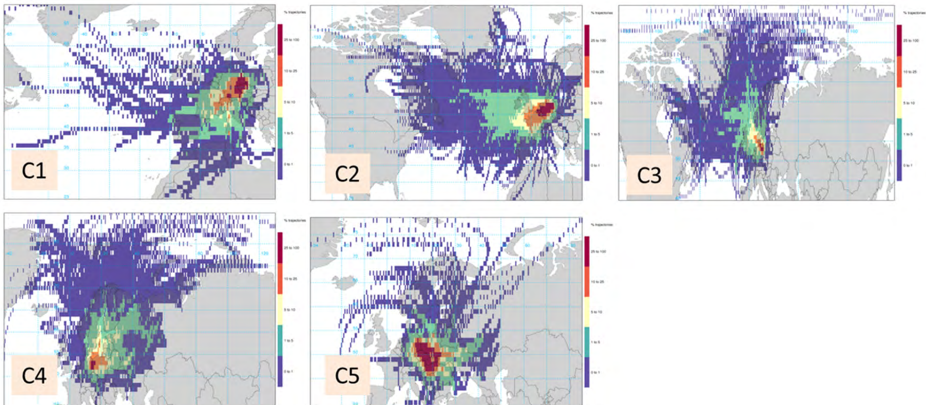
Abbildung 41: Überströmte Gebiete in Europa, Trajektorien ausgehend von BEFRA in den Clustern C1 bis C5 (vgl. auch Abbildung 40)
