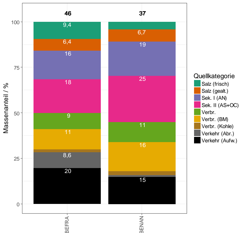
Abbildung 61: Anteile der auf PMF Level 5 identifizierten Quellkategorien an der mittleren PM10- Massekonzentration (schwarze Zahlen über Balken) der beiden Berliner Stationen.
