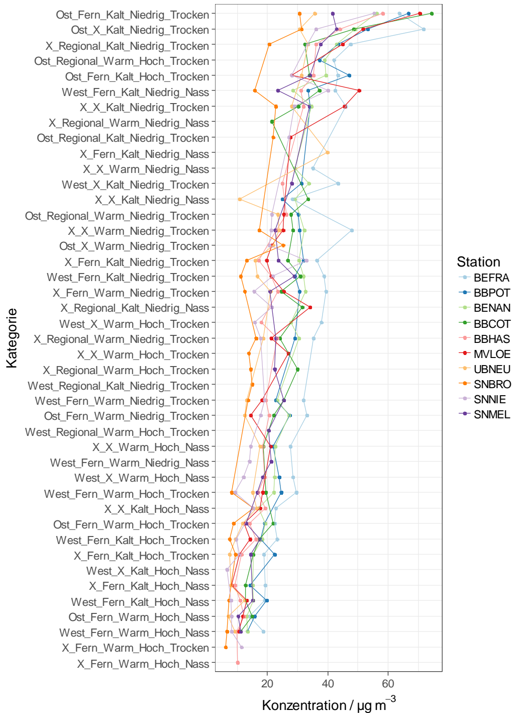
Abbildung 38: Mittlere Konzentrationen an PM10 für die einzelnen Stationen in den kombinierten Kategorien. Die kombinierten Kategorien sind nach Größe der PM10- Massekonzentration sortiert.
