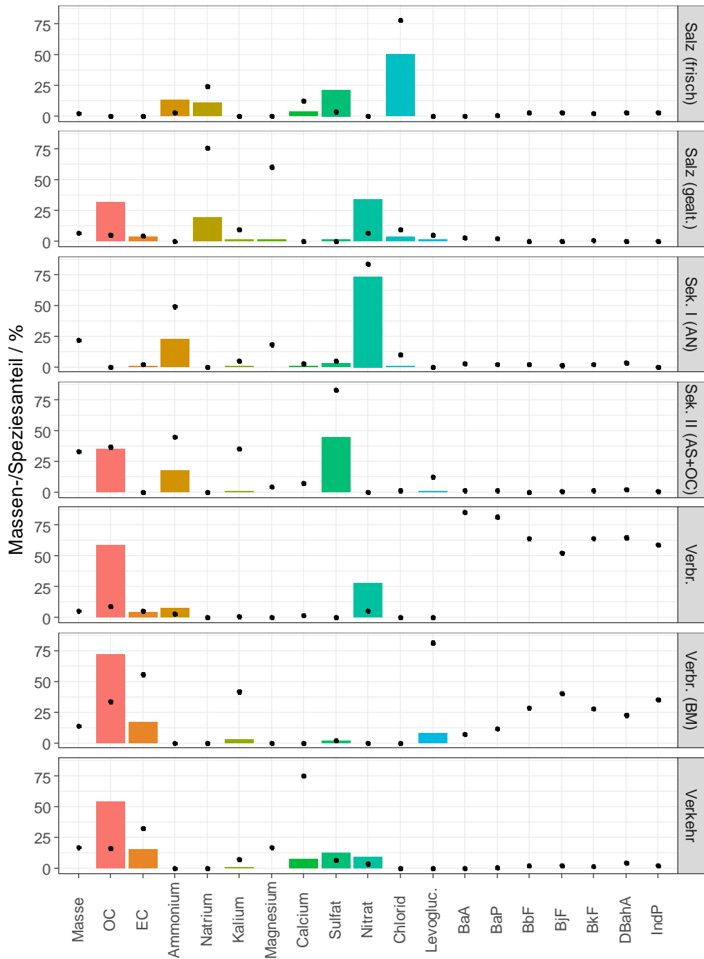
Abbildung 48: Quellprofile der 7 Faktoren des Level 4 PMF Laufes. Balken geben den Massenanteil in % der Faktormasse an (Summe aller Verbindungen im Faktor = 100%), Punkte den Speziesanteil in % der Gesamt-Spezieskonzentration (Summe der Spezies über alle Faktoren = 100%).
