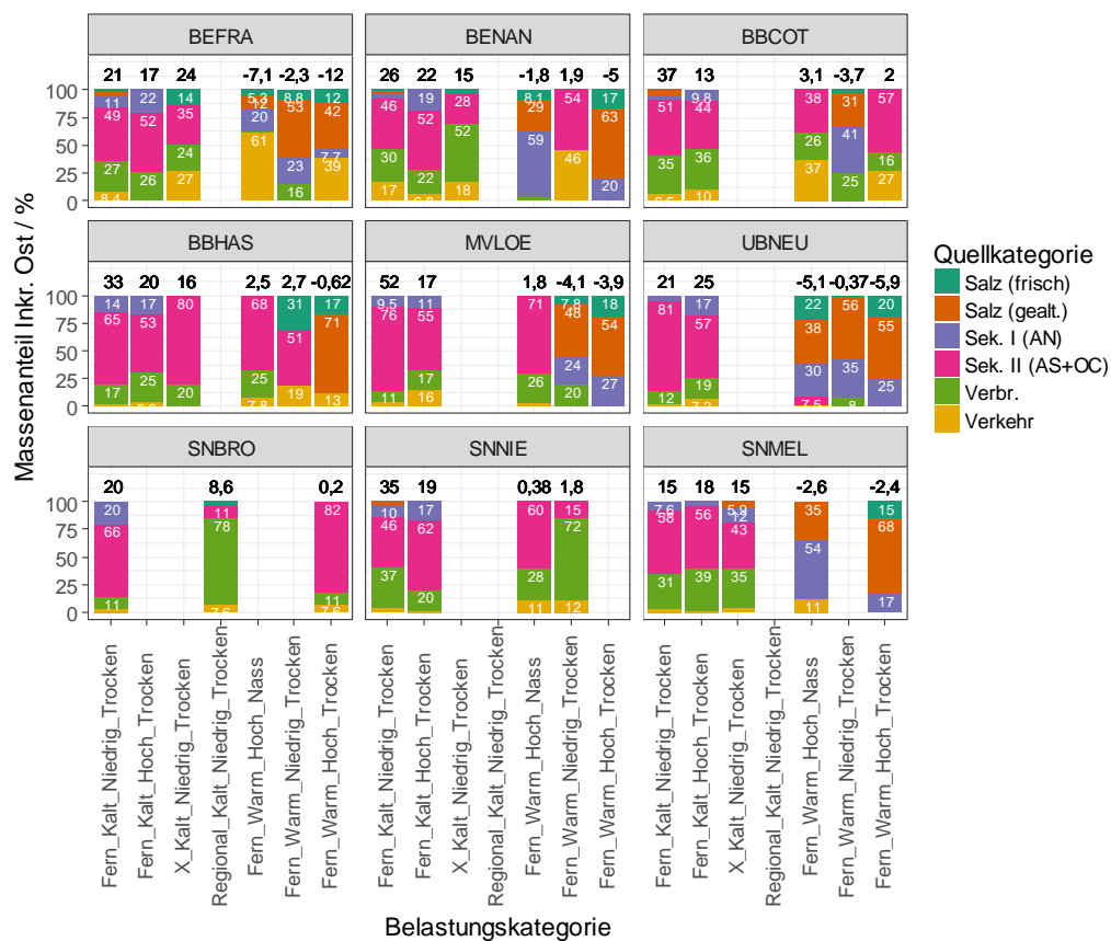
Abbildung 68: Massenanteil Inkrement Ost in % der Quellkategorien am „Netto“- Inkrement- Ost (schwarze Zahlen über Säulen in \mu\text{g m}^{-3} ) in Abhängigkeit von den kombinierten Belastungskategorien, dargestellt für alle 9 Messstation aus Level 1.
