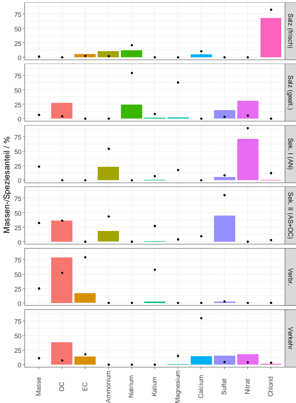
Abbildung 46: Quellprofile der 6 Faktoren des Level 2 PMF Laufes. Balken geben den Massenanteil in % der Faktormasse an (Summe aller Verbindungen im Faktor = 100%), Punkte den Speziesanteil in % der Gesamt-Spezieskonzentration (Summe der Spezies über alle Faktoren = 100%).
