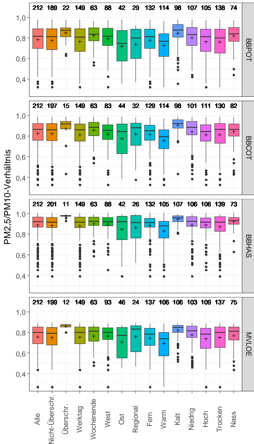
Abbildung 25: Verhältnis der PM 2,5 / PM 10 - Massekonzentration für „Alle“ Messtage, in Abhängigkeit von der Tagescharakteristik und den Belastungskategorien für die Messstationen BBPOT, BBCOT, BBHAS und MVLOE. Die Zahlen über den Boxen kennzeichnen die Anzahl der verfügbaren Messtage.
