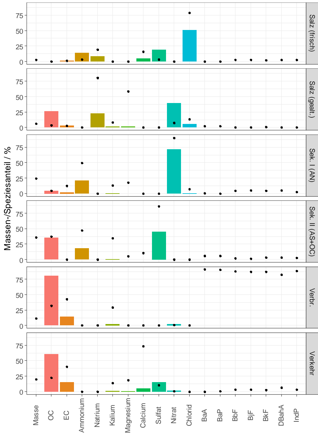
Abbildung 47: Quellprofile der 6 Faktoren des Level 3 PMF Laufes. Balken geben den Massenanteil in % der Faktormasse an (Summe aller Verbindungen im Faktor = 100%), Punkte den Speziesanteil in % der Gesamt-Spezieskonzentration (Summe der Spezies über alle Faktoren = 100%).
