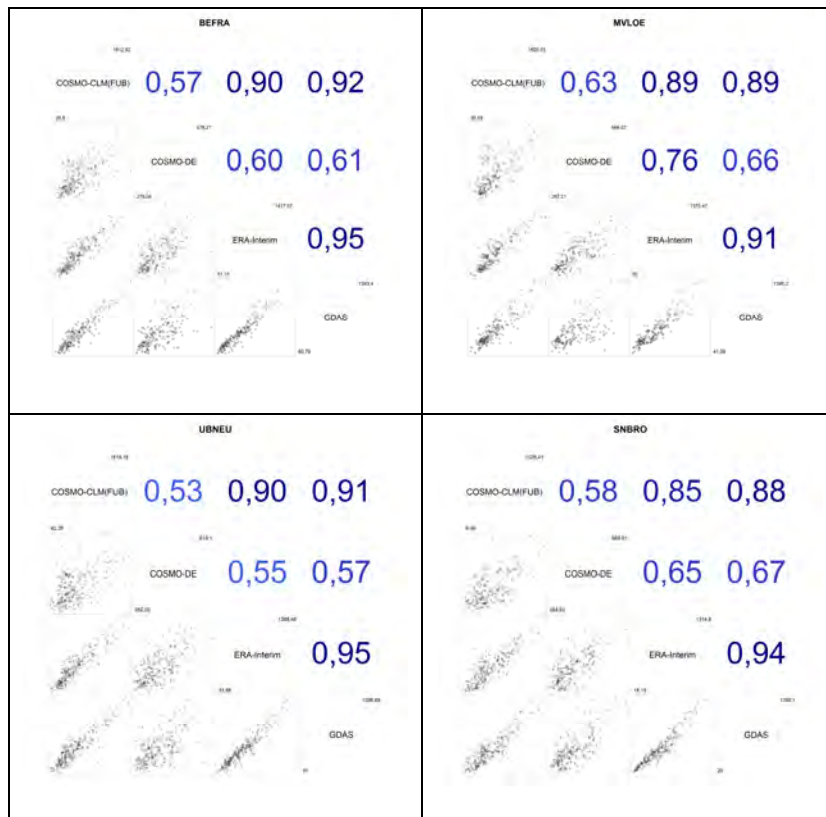
Abbildung 8: Korrelationsmatrizen für die verschiedenen Versionen der Mischungsschichthöhe an 4 ausgewählten Stationen.
