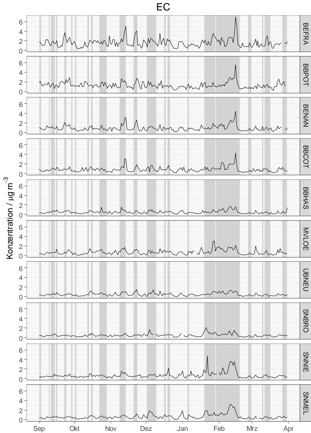
Abbildung 17: Tägliche Konzentration von EC im PM10 für die einzelnen Messstationen im Untersuchungszeitraum; SMT grau hinterlegt.
