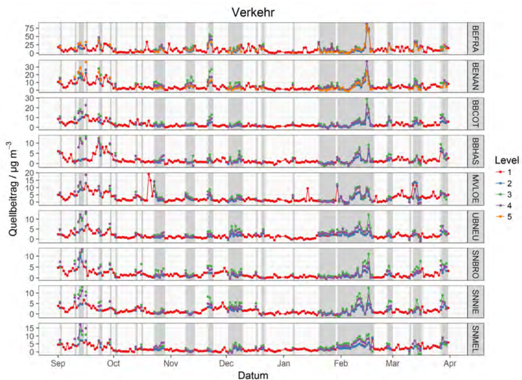
Abbildung 56: Zeitreihen der PMF-modellierten Quellbeiträge für den Faktor Verkehr im direkten Vergleich der 5 PMF Levels.
