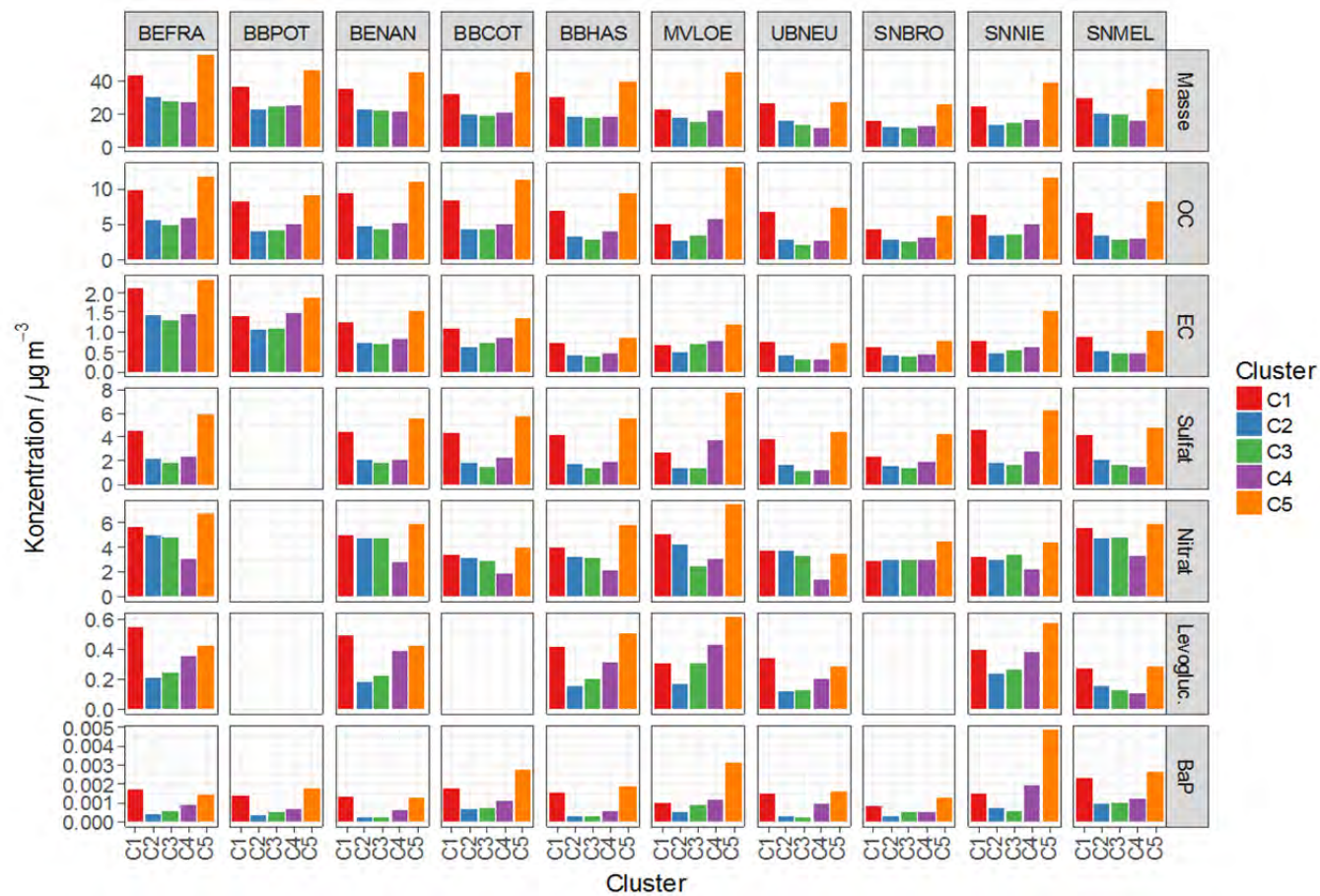
Abbildung 43: Mittlere Konzentrationen in den Clustern C1-C5 im Untersuchungszeitraum, gezeigt für alle Stationen für PM10- Massenkonzentration und die Hauptinhaltsstoffe.
