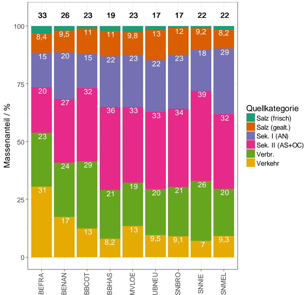
Abbildung 58: Anteile der auf PMF- Level 1 identifizierten Quellkategorien an der mittleren PM10- Massekonzentration (schwarze Zahlen über Balken) der Stationen.
