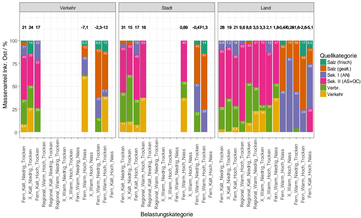
Abbildung 69: Massenanteil Inkrement Ost in % der Quellkategorien am „Netto“- Inkrement- Ost (schwarze Zahlen über Säulen in µg m -3 ) in Abhängigkeit von den kombinierten Belastungskategorien, dargestellt für die Stationstypen Verkehr (= BEFRA), Stadt und Land.
