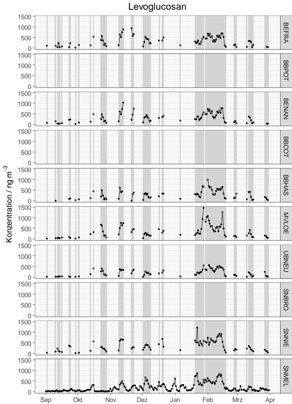
Abbildung 22: Tägliche Konzentration von Levoglucosan im PM10 für die einzelnen Messstationen im Untersuchungszeitraum; SMT grau hinterlegt.
