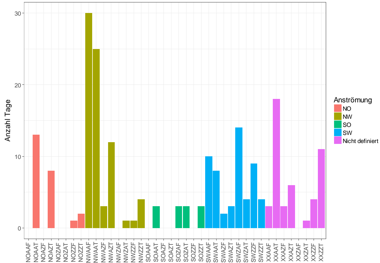
Abbildung 11: Anzahl der Messtage in den Wetterlagenklassen nach OWTC und Eingruppierung nach dem Windindex für 700 hPa.
