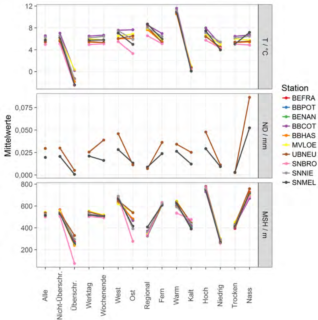
Abbildung 36: Mittelwerte der Parameter T, ND und MSH für alle Messstationen in Abhängigkeit von der Tagescharakteristik und der Belastungskategorie.
