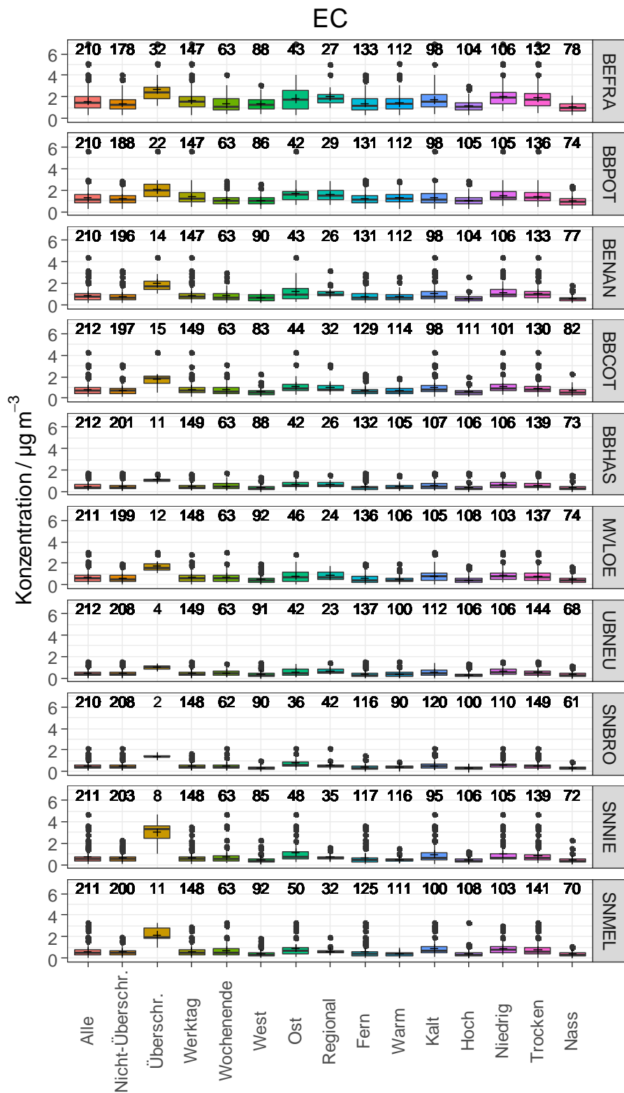
Abbildung 27: EC für „Alle“ Messtage und in Abhängigkeit von der Tagescharakteristik und den Belastungskategorien für alle 10 Messstationen. Die Zahlen über den Boxen kennzeichnen die Anzahl der verfügbaren Messwerte.
