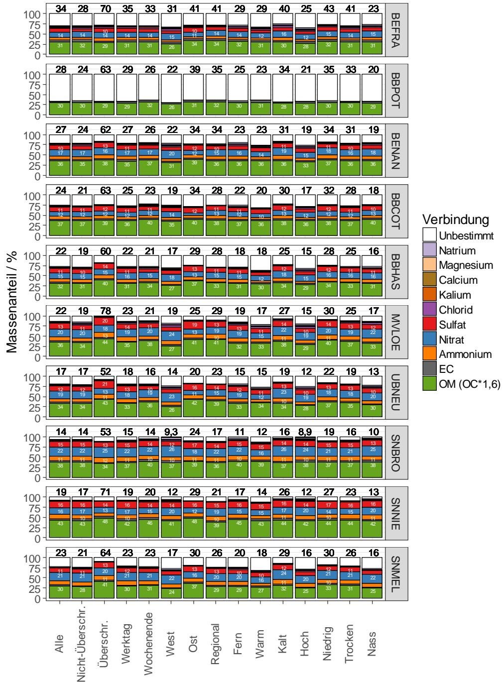
Abbildung 32: Massenbilanz für alle Messtage, in Abhängigkeit von der Tagescharakteristik und den Belastungskategorien. Massenanteile < 10% sind nicht als Zahl angegeben, die schwarzen Zahlen stehen für die mittleren Konzentrationen in \mu\text{g m}^{-3} . OC wurde zu OM mit dem Faktor 1,6 konvertiert.
