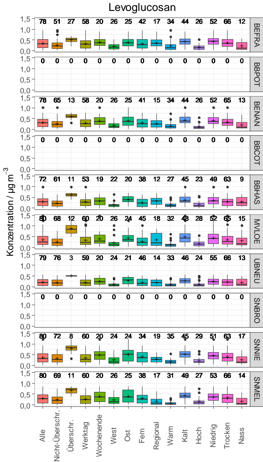
Abbildung 30: Levoglucosan für „Alle“ Sondermesstage und in Abhängigkeit von der Tagescharakteristik und den Belastungskategorien für alle 10 Messstationen. Die Zahlen über den Boxen kennzeichnen die Anzahl der verfügbaren Messwerte.
