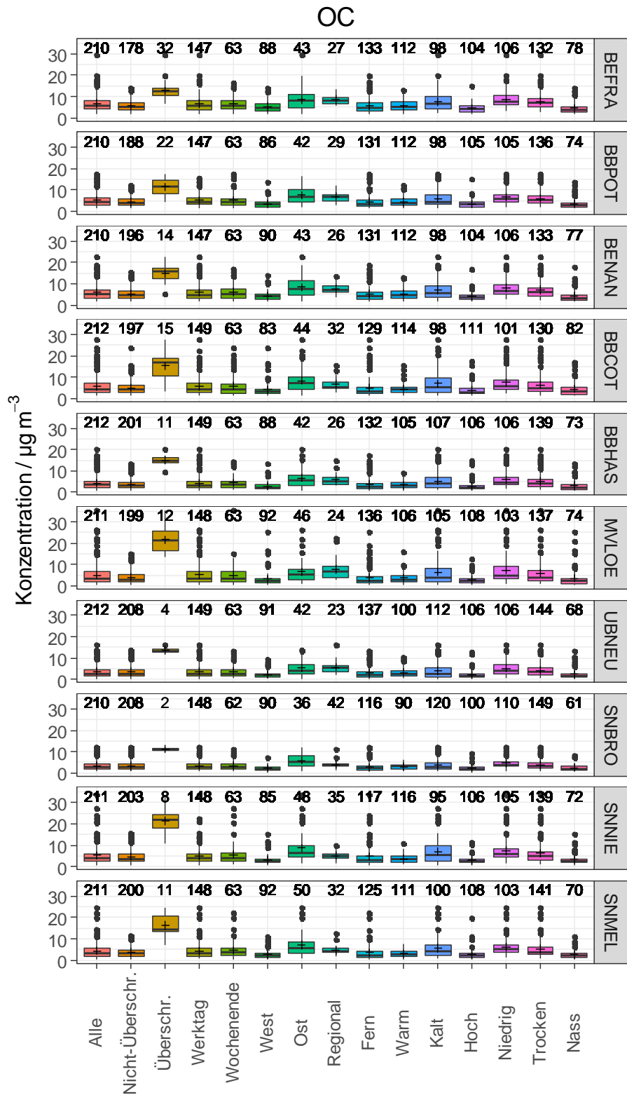
Abbildung 26: OC für „Alle“ Messtage und in Abhängigkeit von der Tagescharakteristik und den Belastungskategorien für alle 10 Messstationen. Die Zahlen über den Boxen kennzeichnen die Anzahl der verfügbaren Messwerte.
