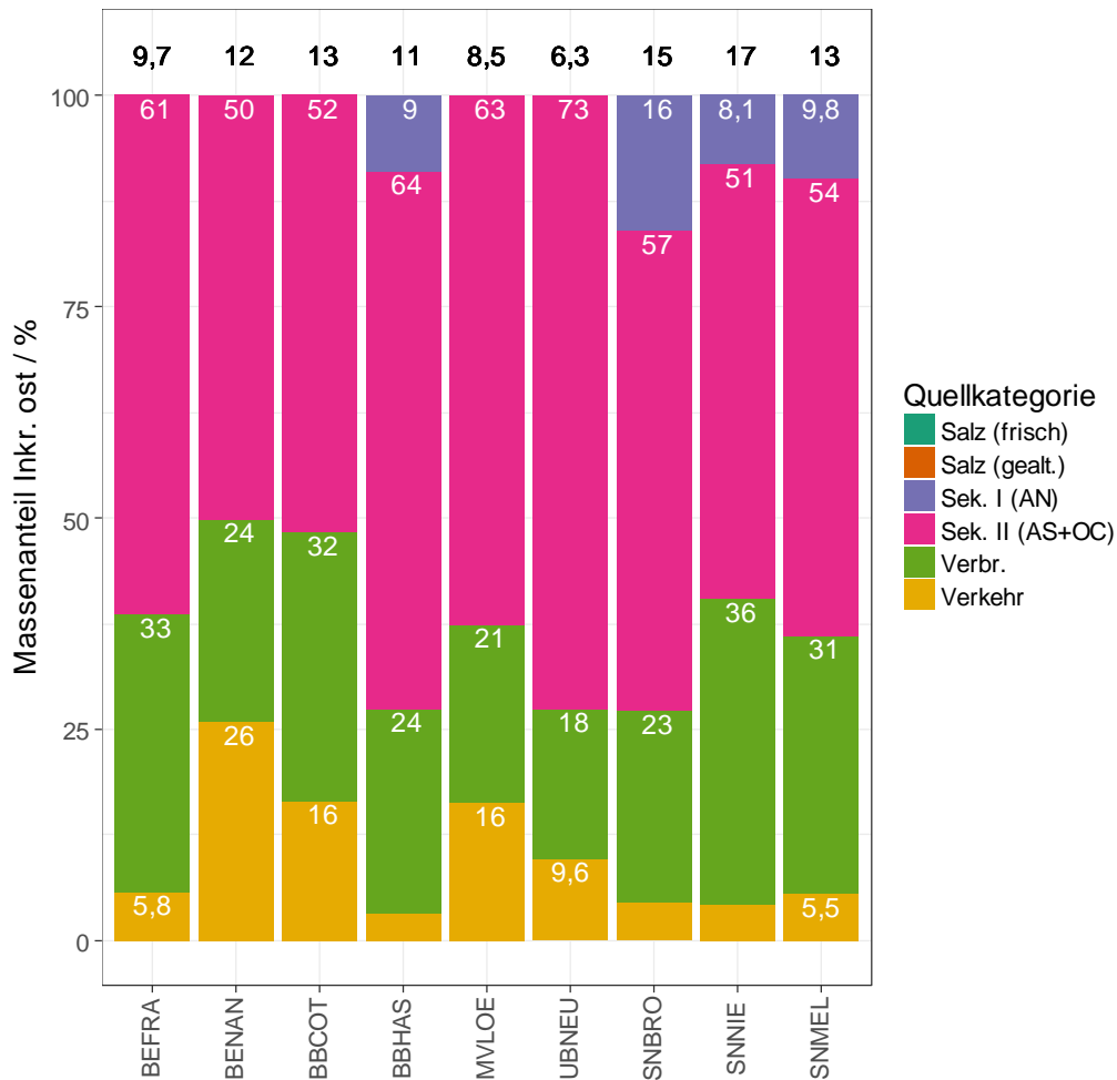
Abbildung 67: Massenanteil Inkrement Ost in % der Quellkategorien am „Netto“- Inkrement- Ost (schwarze Zahlen über Säulen in \mu\text{g m}^{-3} ) dargestellt für alle 9 Messstation aus Level 1.
