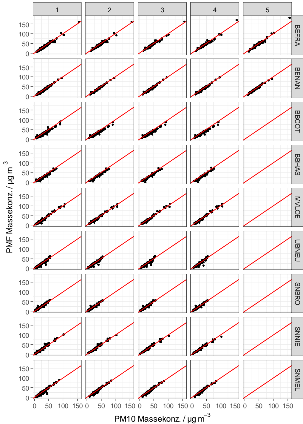
Abbildung 57: Vergleich der gemessenen PM10- Massekonzentration mit der durch PMF zugeordneten Konzentration an allen Stationen und für alle PMF Levels (Spalten). Die rote Linie zeigt die 1:1 Gerade.
