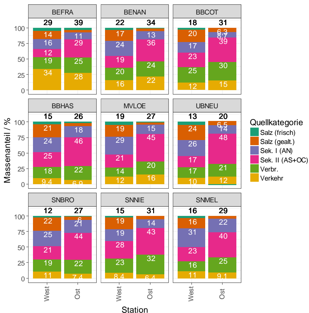
Abbildung 65: Massenannteile der Quellkategorien für die aus der PMF resultierenden PM10- Massekonzentration (schwarze Zahlen über Säulen in \mu\text{g m}^{-3} ) in Abhängigkeit von der Anströmung, dargestellt für alle 9 Messstation aus Level 1.
