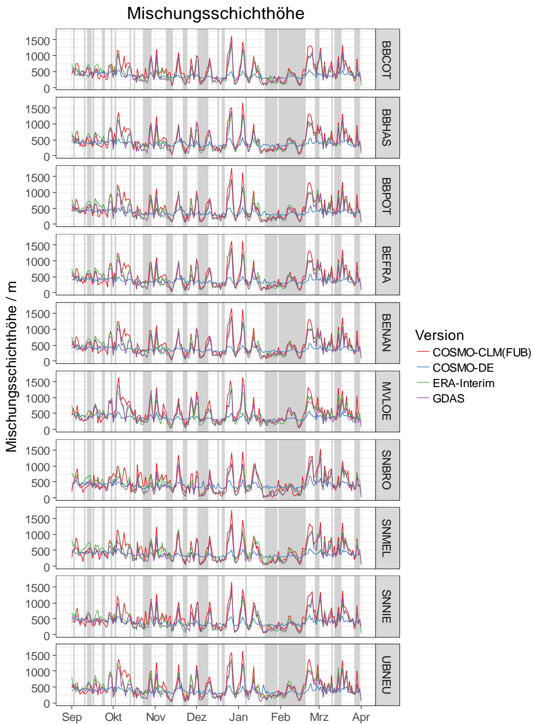
Abbildung 7: Tagesmittel der Mischungsschichthöhe für jede Messstation im Untersuchungszeitraum; SMT grau hinterlegt.
