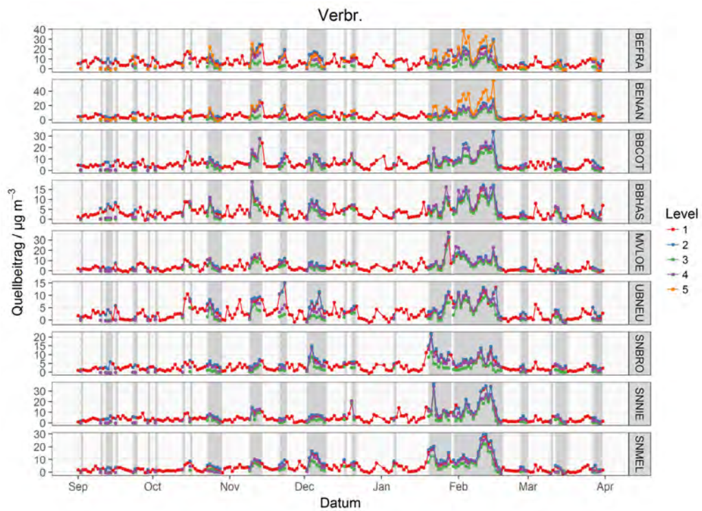
Abbildung 55: Zeitreihen der PMF-modellierten Quellbeiträge für den Faktor Verbrennung im direkten Vergleich der 5 PMF Levels.
