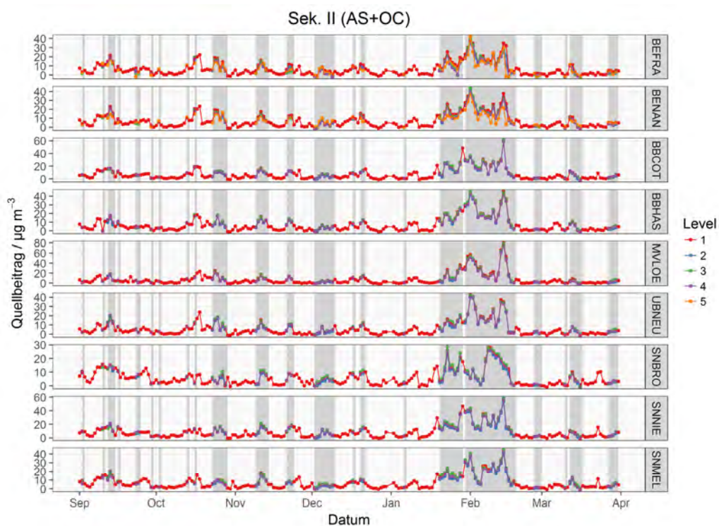
Abbildung 54: Zeitreihen der PMF-modellierten Quellbeiträge für den sek. Quellfaktor II (AS+OC) im direkten Vergleich der 5 PMF Levels.
