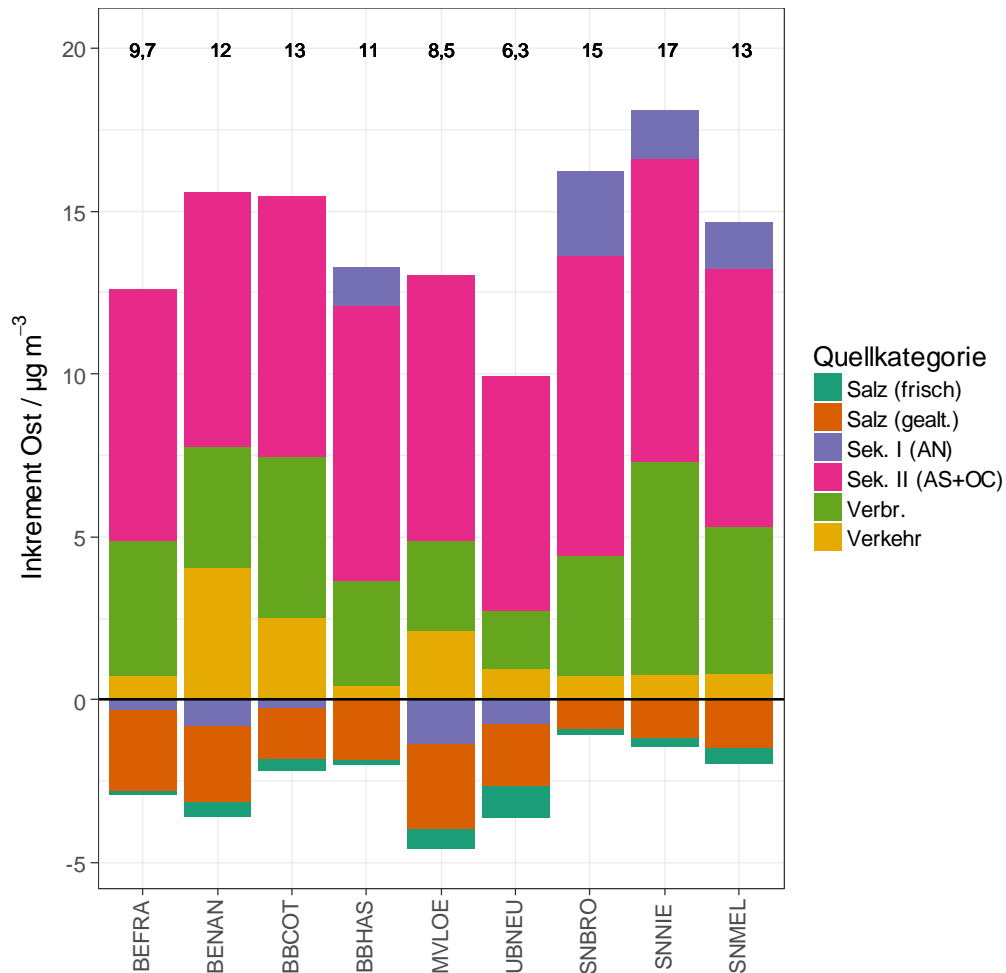
Abbildung 66: Inkrement Ost der Quellkategorien (schwarze Zahlen über Säulen in \mu\text{g m}^{-3} ) für die aus der PMF resultierenden PM10- Massekonzentrationen dargestellt für alle 9 Messstation aus Level 1.
