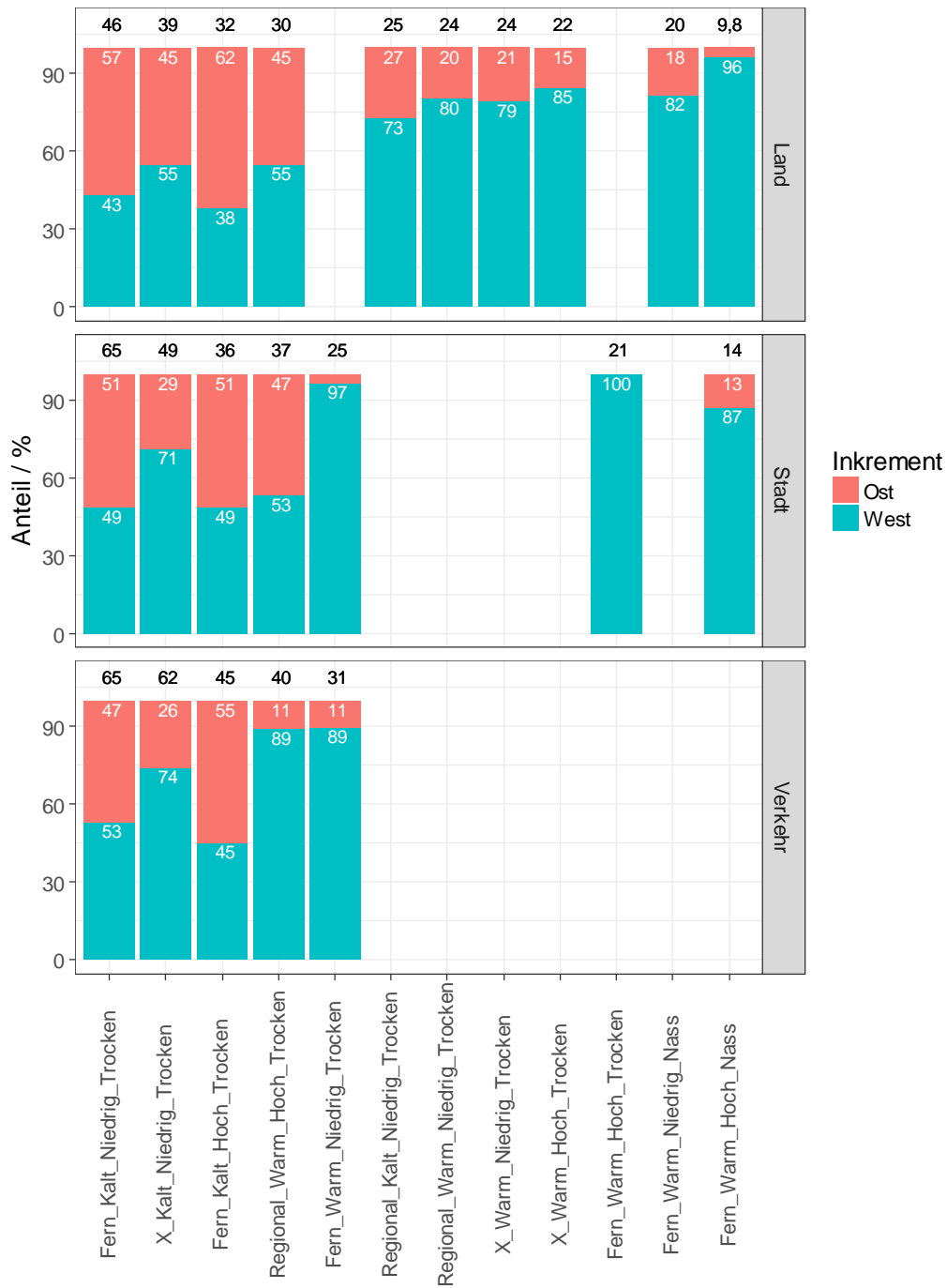
Abbildung 39: Mittlere Beiträge des grenzüberschreitenden Ferneintrages von PM10 aus östlicher Richtung ins Untersuchungsgebiet (Inkrement Ost). Schwarze Zahlen über den Balken geben die mittlere Konzentration bei Ostanströmung in \mu\text{g m}^{-3} an, weiße Zahlen die Anteile des Hintergrundniveaus (West) und des zusätzlich antransportierten Beitrages (Ost) unter den jeweiligen meteorologischen Bedingungen, jeweils gemittelt nach Stationstyp.
