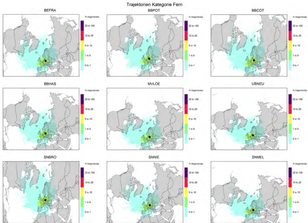
Abbildung 6: Geographische Häufigkeitsverteilungen für 96h- Rückwärtstrajektorien der Kategorie „Fern“ im Untersuchungszeitraum. Auf die Darstellung der Messstation BENAN wurde aufgrund der lokalen Nähe zur Messstation BEFRA verzichtet.
