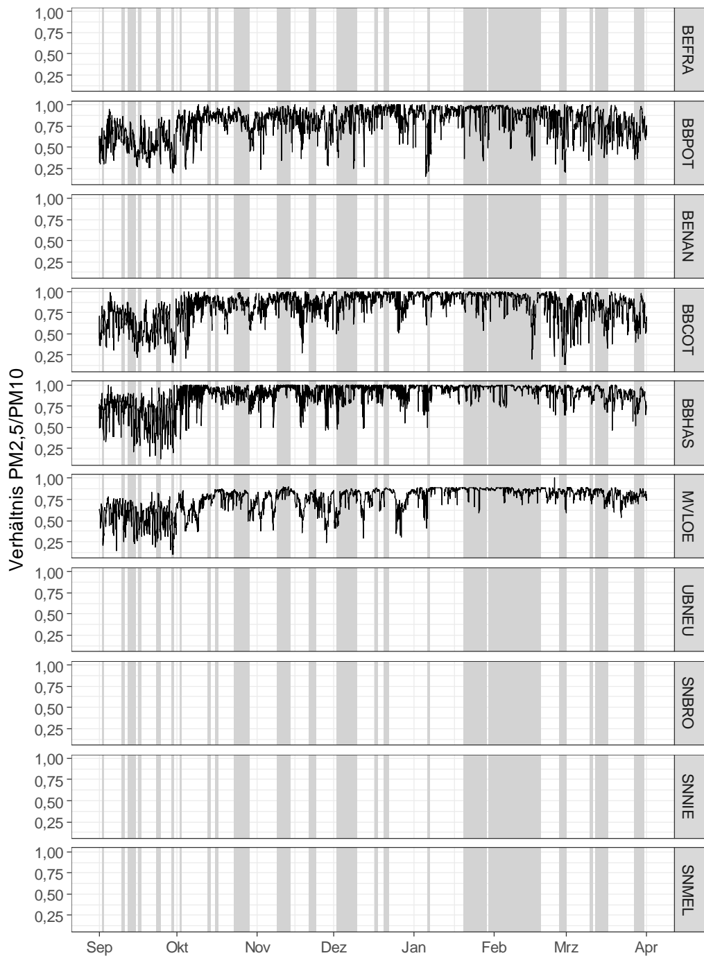
Abbildung 15: Verhältnis PM 2,5 / PM 10 im Untersuchungszeitraum für die einzelnen Messstationen; SMT grau hinterlegt.
