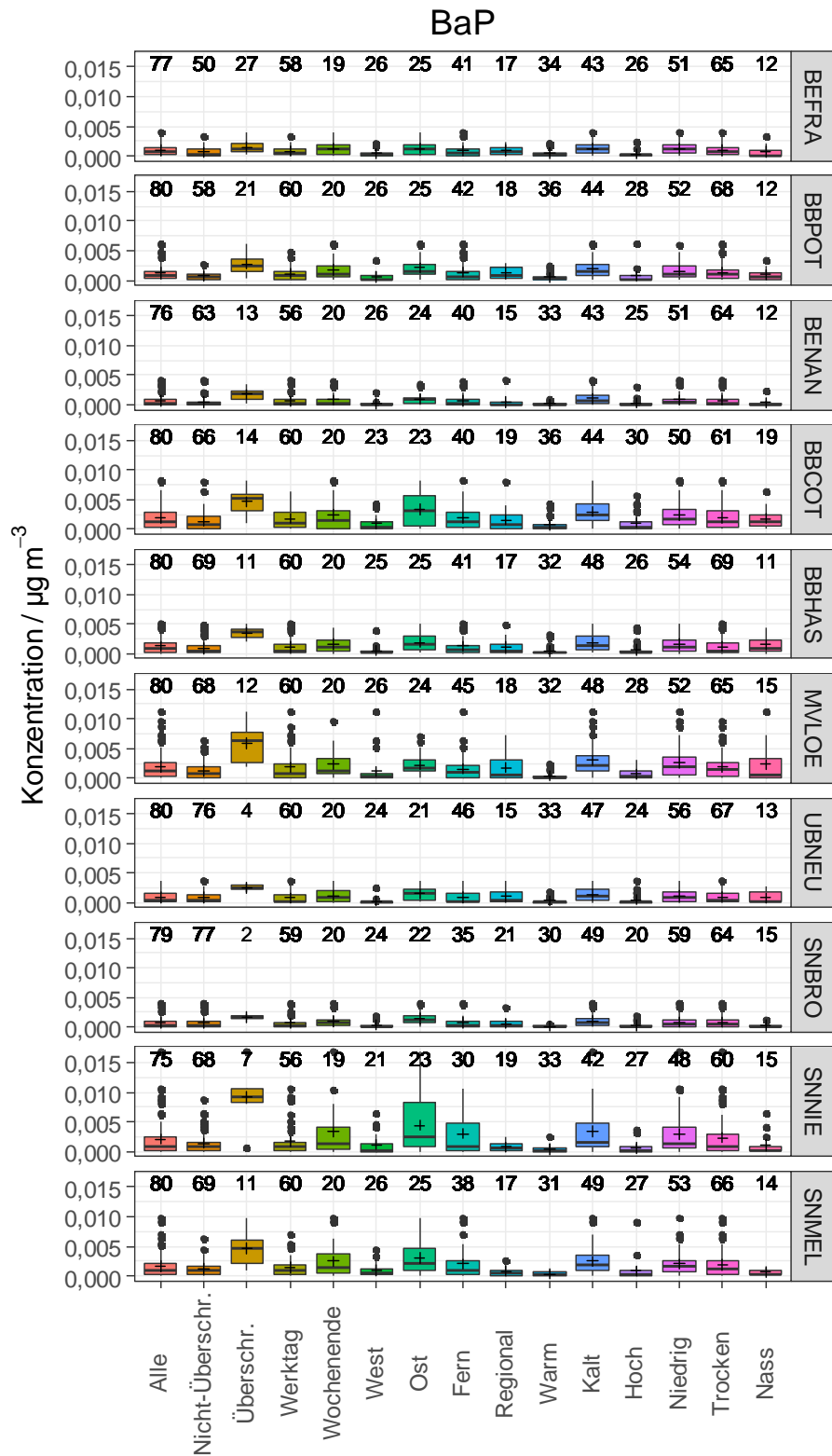
Abbildung 31: BaP für „Alle“ Sondermesstage und in Abhängigkeit von der Tagescharakteristik und den Belastungskategorien für alle 10 Messstationen. Die Zahlen über den Boxen kennzeichnen die Anzahl der verfügbaren Messwerte.
