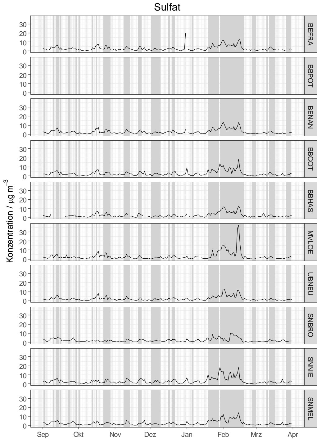
Abbildung 19: Tägliche Konzentration von Sulfat im PM10 für die einzelnen Messstationen im Untersuchungszeitraum; SMT grau hinterlegt.
