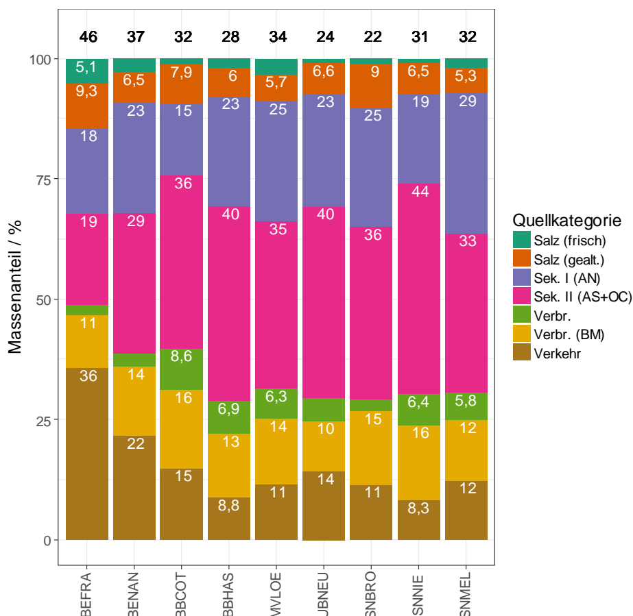
Abbildung 60: Anteile der auf PMF Level 4 identifizierten Quellkategorien an der mittleren PM10- Massekonzentration (schwarze Zahlen über Balken) der Stationen.
