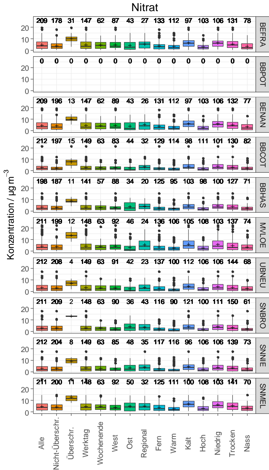
Abbildung 29: Nitrat für „Alle“ Messtage und in Abhängigkeit von der Tagescharakteristik und den Belastungskategorien für alle 10 Messstationen. Die Zahlen über den Boxen kennzeichnen die Anzahl der verfügbaren Messwerte.
