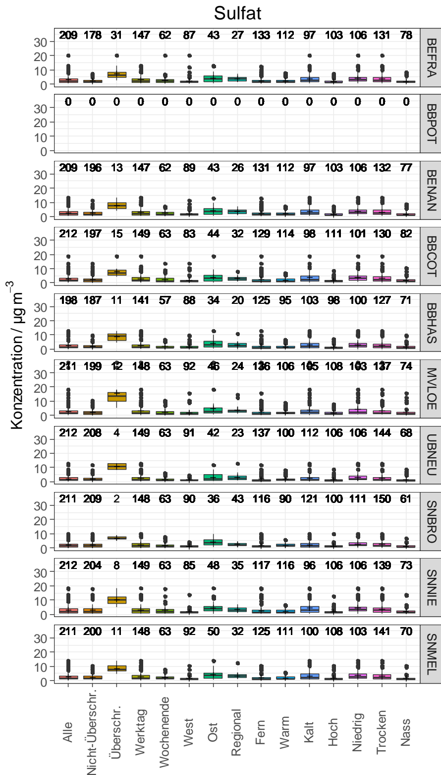
Abbildung 28: Sulfat für „Alle“ Messtage und in Abhängigkeit von der Tagescharakteristik und den Belastungskategorien für alle 10 Messstationen. Die Zahlen über den Boxen kennzeichnen die Anzahl der verfügbaren Messwerte.
