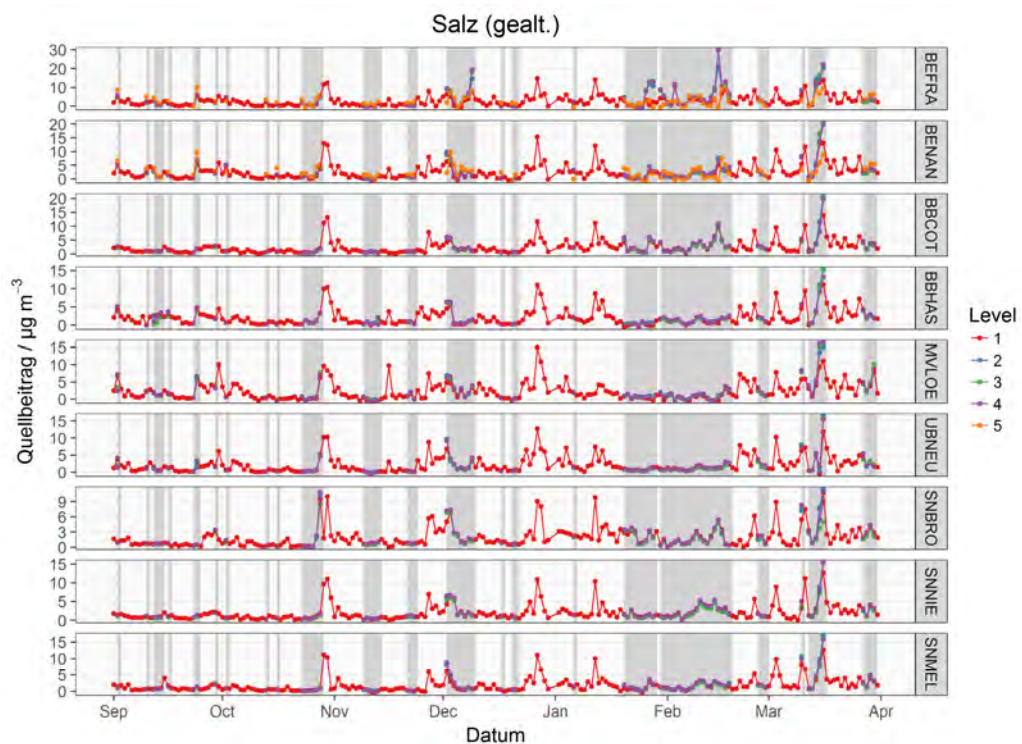
Abbildung 52: Zeitreihen der PMF-modellierten Quellbeiträge für den Faktor gealtertes Salz im direkten Vergleich der 5 PMF Levels.
