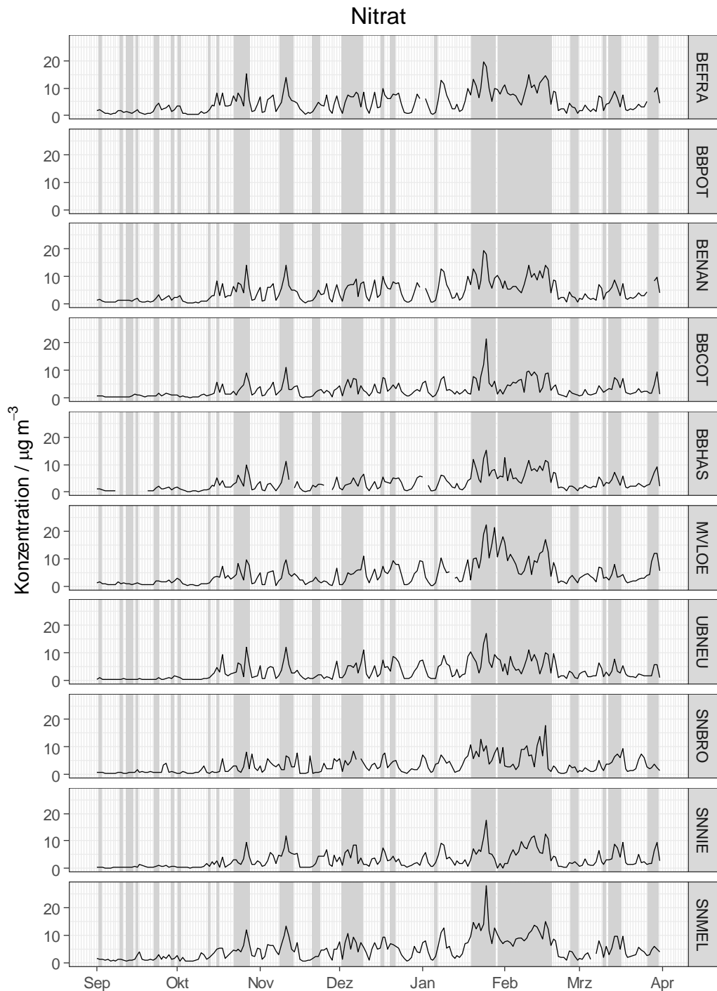
Abbildung 21: Tägliche Konzentration von Nitrat im PM10 für die einzelnen Messstationen im Untersuchungszeitraum; SMT grau hinterlegt.
