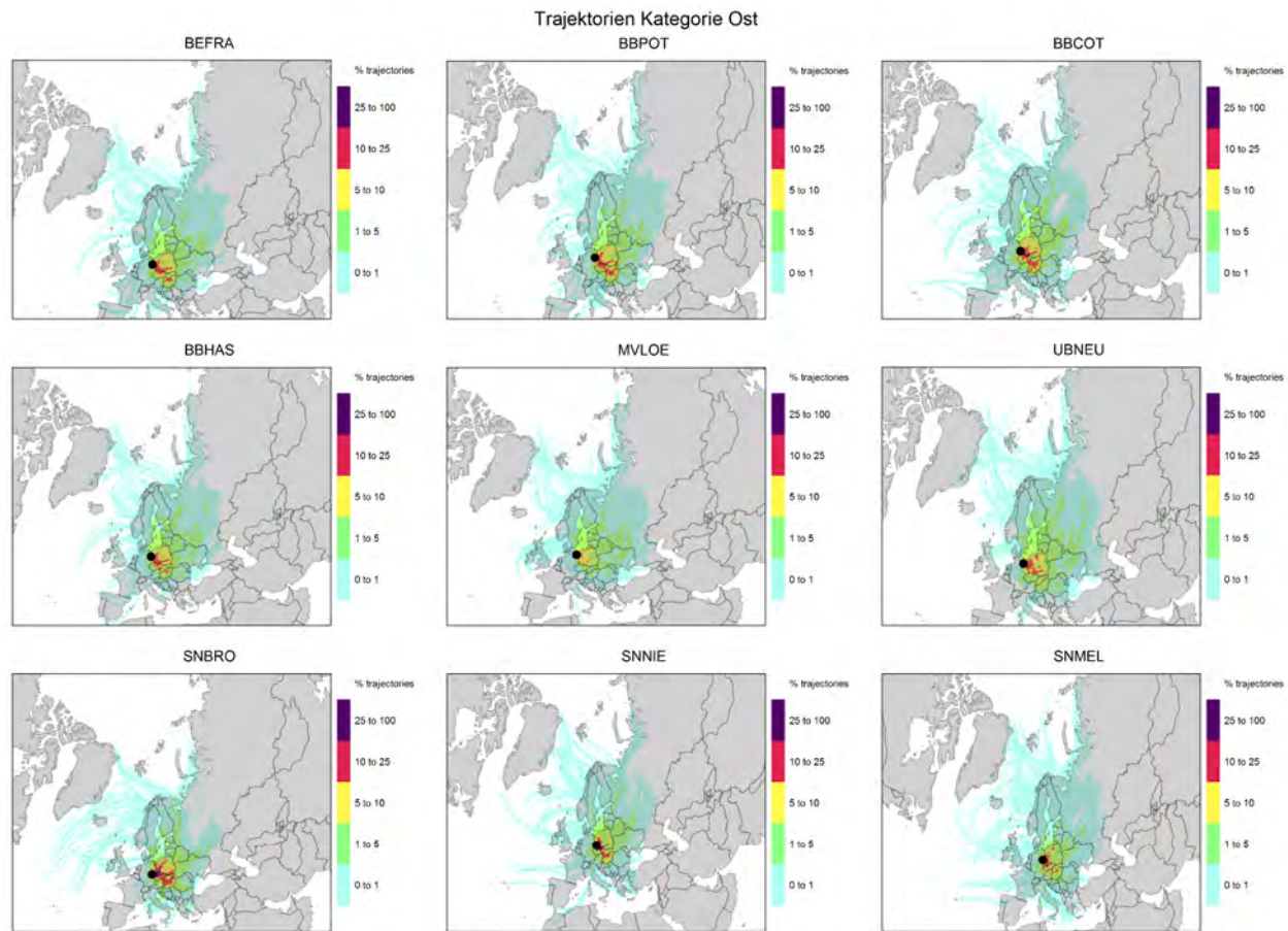
Abbildung 4: Geographische Häufigkeitsverteilung für 96h- Rückwärtstrajektorien der Kategorie „Ost“ im Untersuchungszeitraum. Auf die Darstellung der Messstation BENAN wurde aufgrund der lokalen Nähe zur Messstation BEFRA verzichtet.
