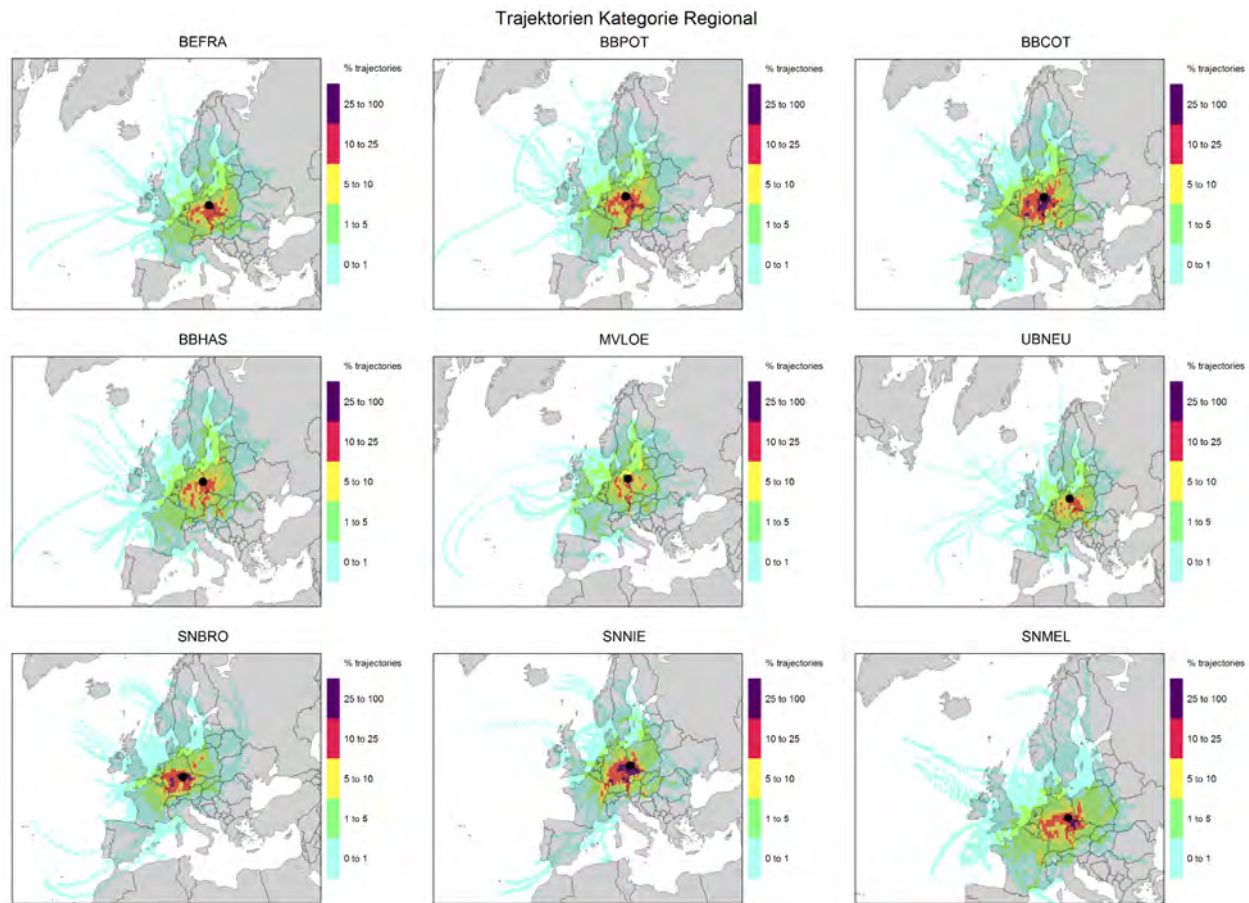
Abbildung 5: Geographische Häufigkeitsverteilung für 96h-Rückwärtstrajektorien der Kategorie „Regional“ im Untersuchungszeitraum. Auf die Darstellung der Messstation BENAN wurde aufgrund der lokalen Nähe zur Messstation BEFRA verzichtet.
