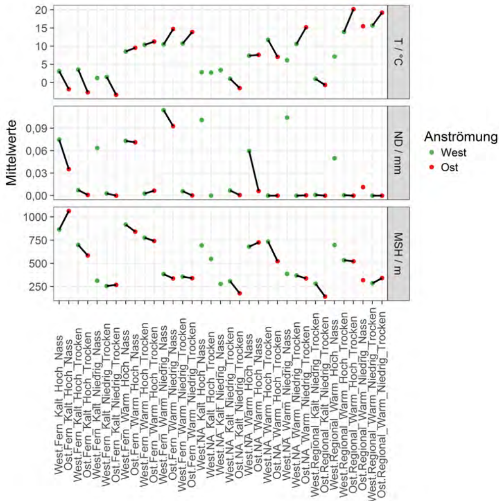
Abbildung 37: Mittelwerte der Parameter T, ND und MSH für die 6 ländlichen Hintergrundstationen in Abhängigkeit von der Anströmung („West“ vs. „Ost“) in den kombinierten Belastungskategorien.
