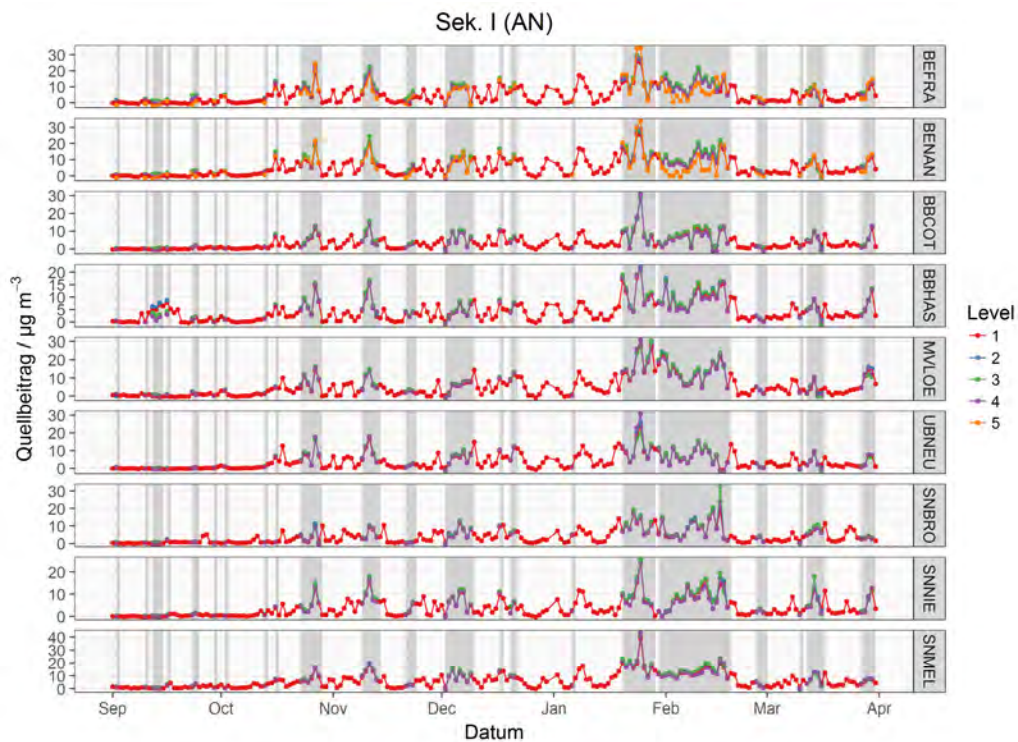
Abbildung 53: Zeitreihen der PMF-modellierten Quellbeiträge für den sek. Quellfaktor I (AN) im direkten Vergleich der 5 PMF Levels.
