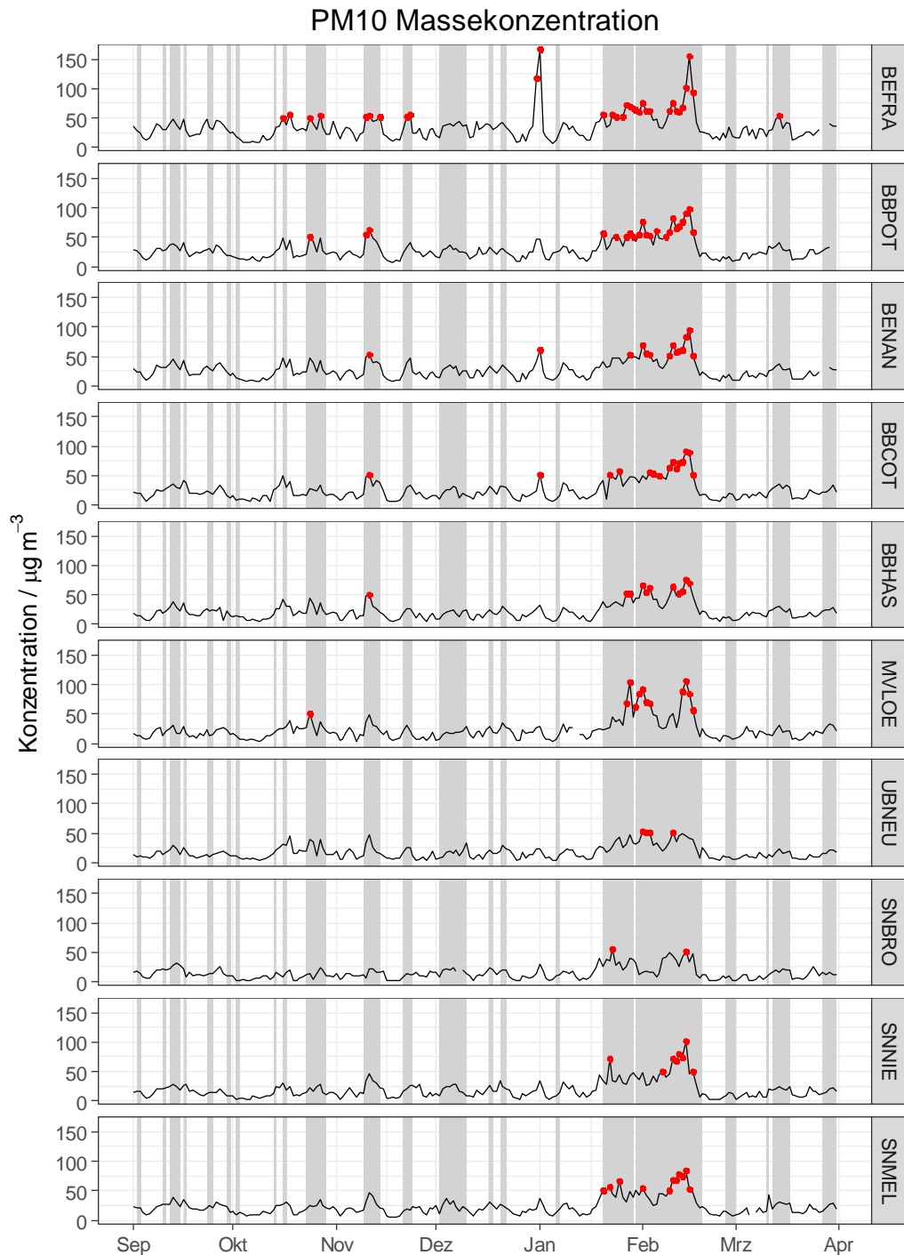
Abbildung 13: Tägliche PM10- Massekonzentrationen für alle Messstationen im Untersuchungszeitraum; rote Punkte markieren Grenzwert-Überschreitungstage; SMT grau hinterlegt.
