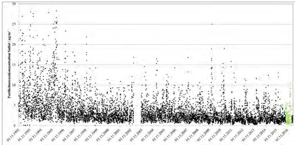
Abbildung 20: Verlauf der täglichen Sulfatkonzentration in PM10 an der Station SNMEL seit 1992. Die Ergebnisse der 212 Tage des PM-OST Projektes sind in grün gezeigt.
