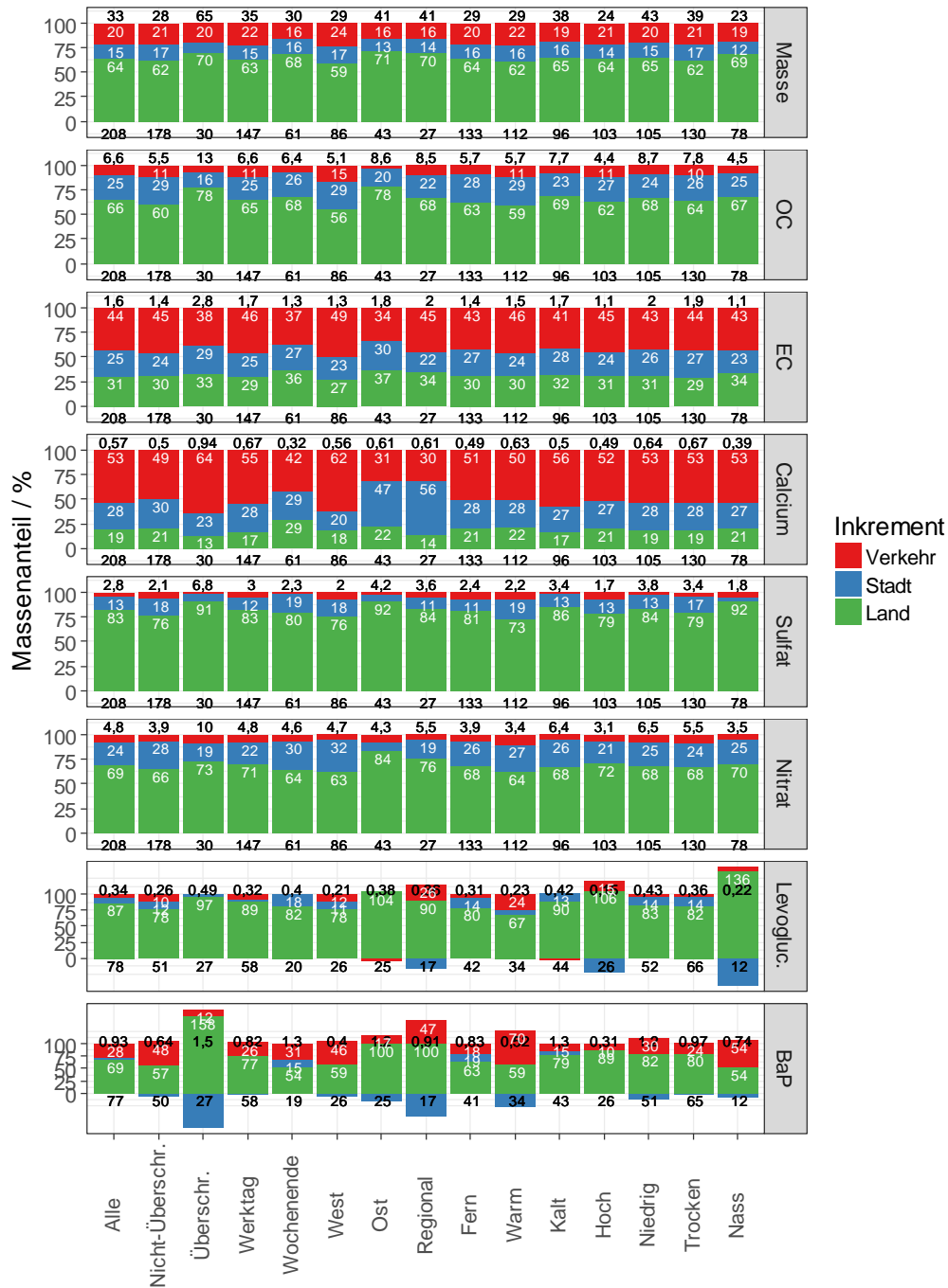
Abbildung 35: Massenanteil PM10 und Inhaltsstoffe der Inkremente Verkehr, Stadt und Land für alle Messtage (Alle) und gruppiert entsprechend der Tagescharakteristik und der Belastungskategorie unter Auswertung der PM10-Masse der Messstationen BEFRA, BENAN und BBHAS im Untersuchungszeitraum. Die schwarzen Zahlen über den Boxen repräsentieren die gemittelte PM10-Massekonzentration an der Verkehrsstation BEFRA in \mu\text{g m}^{-3} , unter den Boxen die Anzahl der Messtage. Die weißen Zahlen in den Säulen geben den berechneten prozentualen Anteil der Inkremente an der Gesamtmasse wieder.
