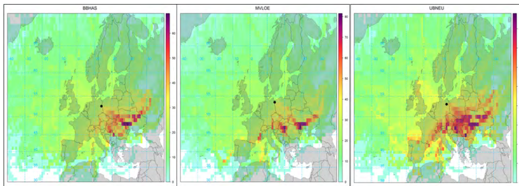
Abbildung 44: CWT- Plots für BBHAS, MVLOE und UBNEU.
