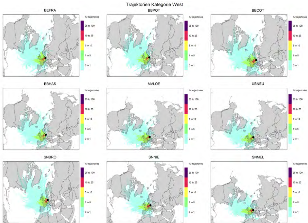
Abbildung 3: Geographische Häufigkeitsverteilung für 96h- Rückwärtstrajektorien der Kategorie „West“ im Untersuchungszeitraum. Auf die Darstellung der Messstation BENAN wurde aufgrund der lokalen Nähe zur Messstation BEFRA verzichtet.
