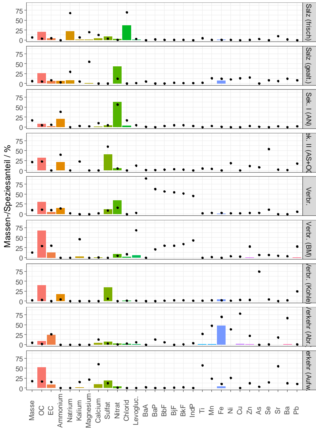
Abbildung 49: Quellprofile der 9 Faktoren des Level 5 PMF Laufes. Balken geben den Massenanteil in % der Faktormasse an (Summe aller Verbindungen im Faktor = 100%), Punkte den Speziesanteil in % der Gesamt-Spezieskonzentration (Summe der Spezies über alle Faktoren = 100%).
