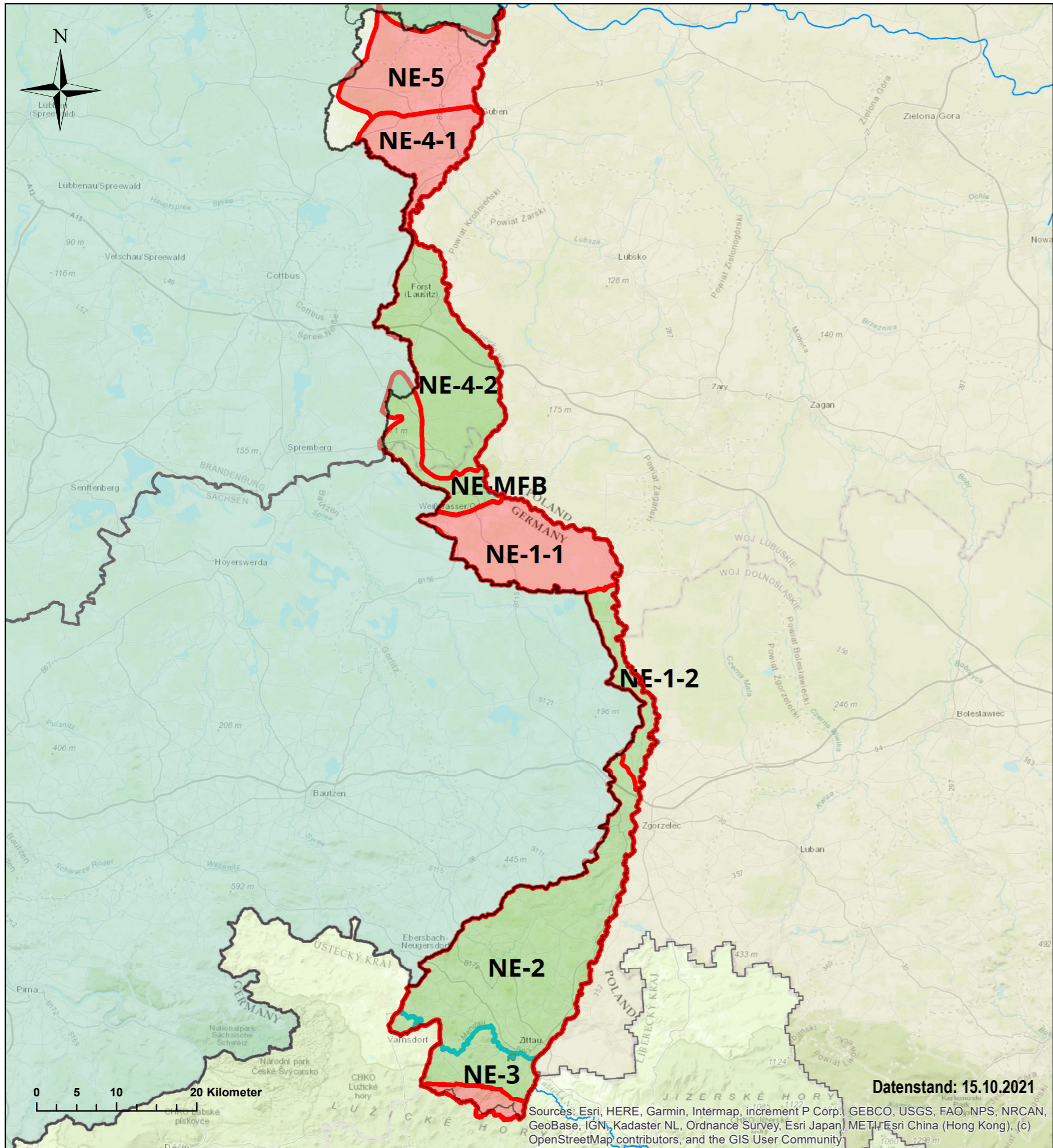
BG LAN - Karte 4.7 - Mengenmäßiger Zustand der Grundwasserkörper
