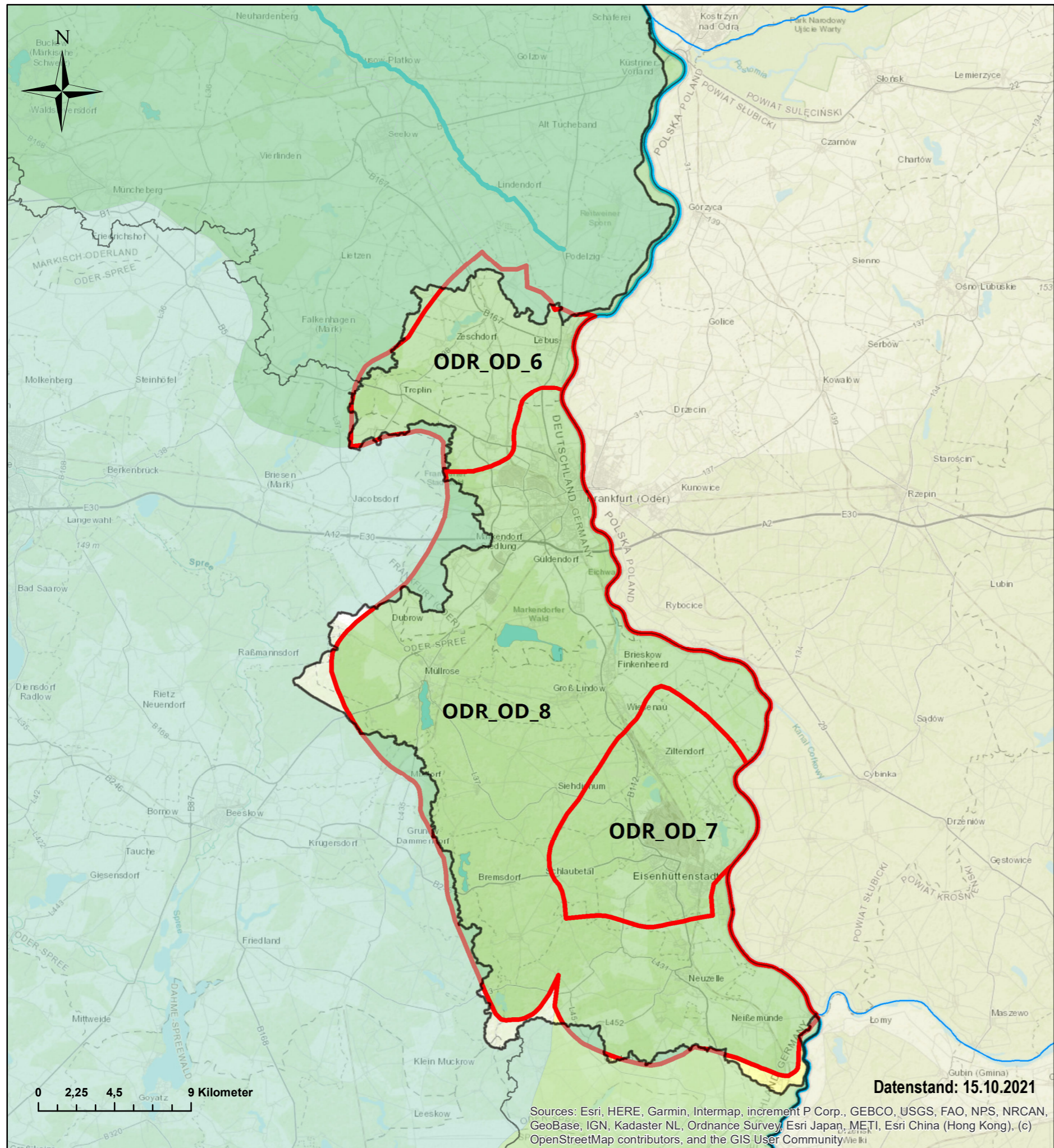
BG MOD - Karte 13.3 - Mengenmäßiger Zustand der Grundwasserkörper - Vergleich 2. und 3. Bewirtschaftungszeitraum
