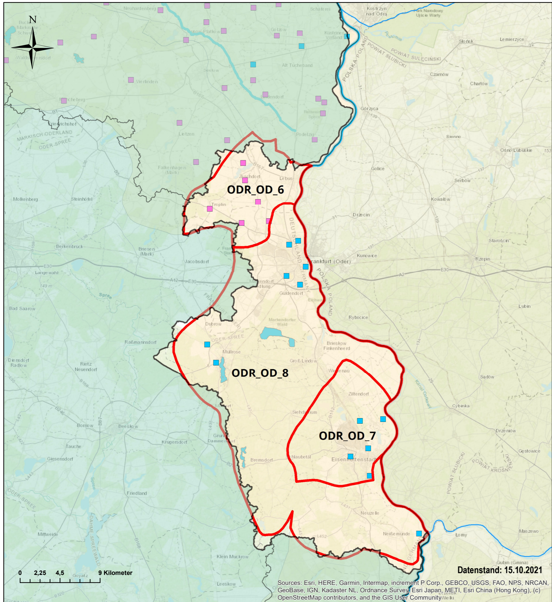
BG MOD - Karte 4.5 - Überwachungsnetz des Grundwassers - Chemie
