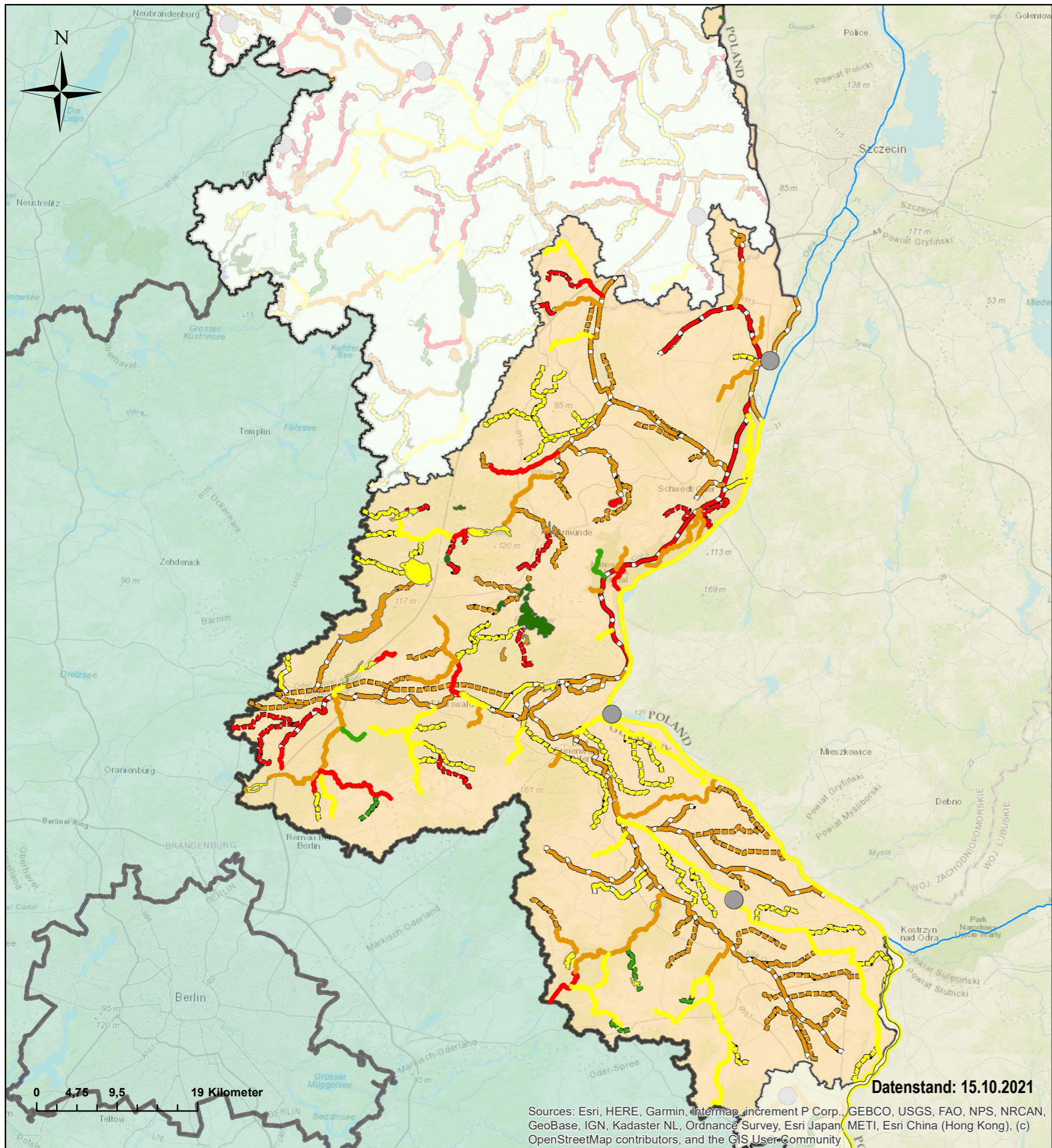
BG UOD - Karte 4.2 - Ökologischer Zustand/Potenzial der Oberflächenwasserkörper
