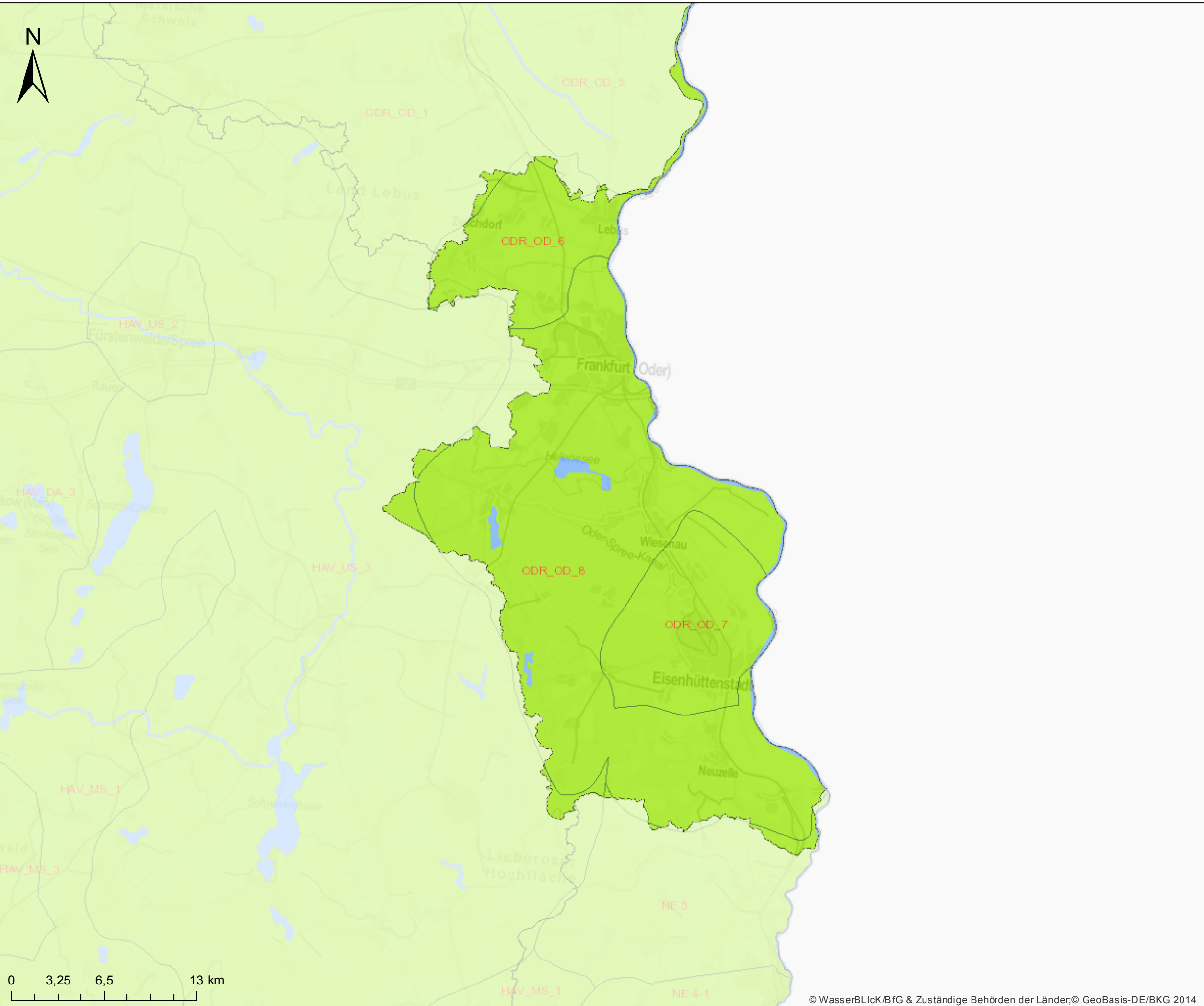
FGE Oder, BG Mittlere Oder, Karte 4.6.2: Chemischer Zustand der Grundwasserkörper hinsichtlich Pestiziden
